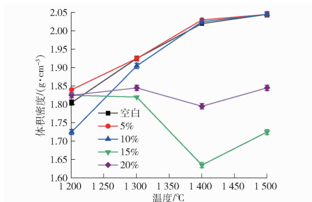
图 4 1 200~1 500 ^{\circ}\text{C} 不同二氧化硅含量对镁铝尖晶石材料影响
