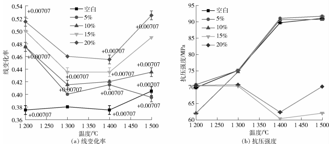
图5 1 200 ~ 1 500 °C 不同二氧化硅含量对镁铝尖晶石材料线变化率和抗压强度影响
