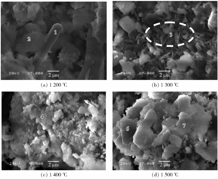
图 7 5% 二氧化硅样品在 1 200 ~1 500 °C 烧结试样粉体 SEM Fig. 7 SEM images of spinel powders with 5% \text{SiO}_2 at 1 200 ~1 500 °C
