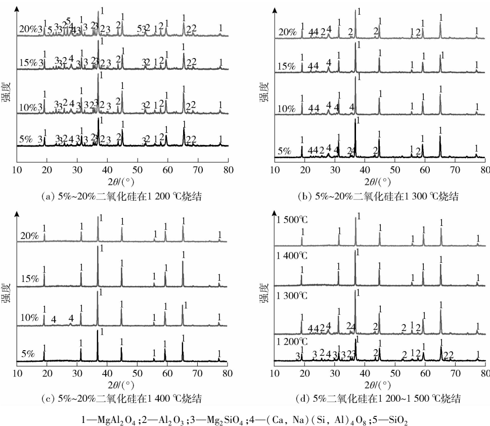
图 6 5% ~20% 二氧化硅在 1 200 ~1 400 °C 烧结 3 h 和 5% 二氧化硅在 1 200 ~1 500 °C 烧结试样 XRD Fig. 6 XRD patterns of spinel with different contents of \text{SiO}_2 at 1 200 ~1 500 °C
