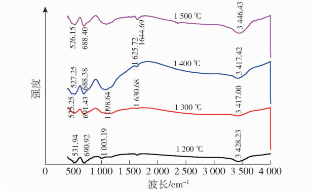
图 8 5% 二氧化硅样品在 1 200 ~ 1 500 °C 烧结材料的 FTIR
