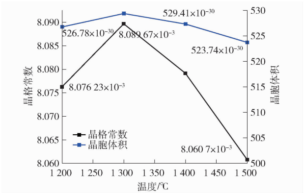
图 9 5% 二氧化硅样品在 1 200 ~ 1 500 °C 烧结镁铝尖晶石晶格常数和晶胞体积
