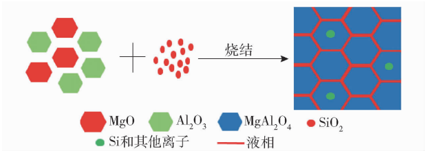
图 10 5% 二氧化硅对材料烧结过程影响示意
