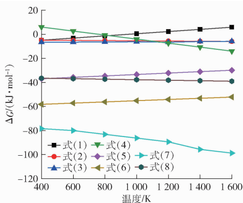
图 3 式(1)~(8)反应吉布斯自由能与温度关系
