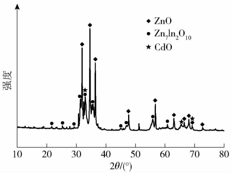
图 10 烟尘 XRD 图
