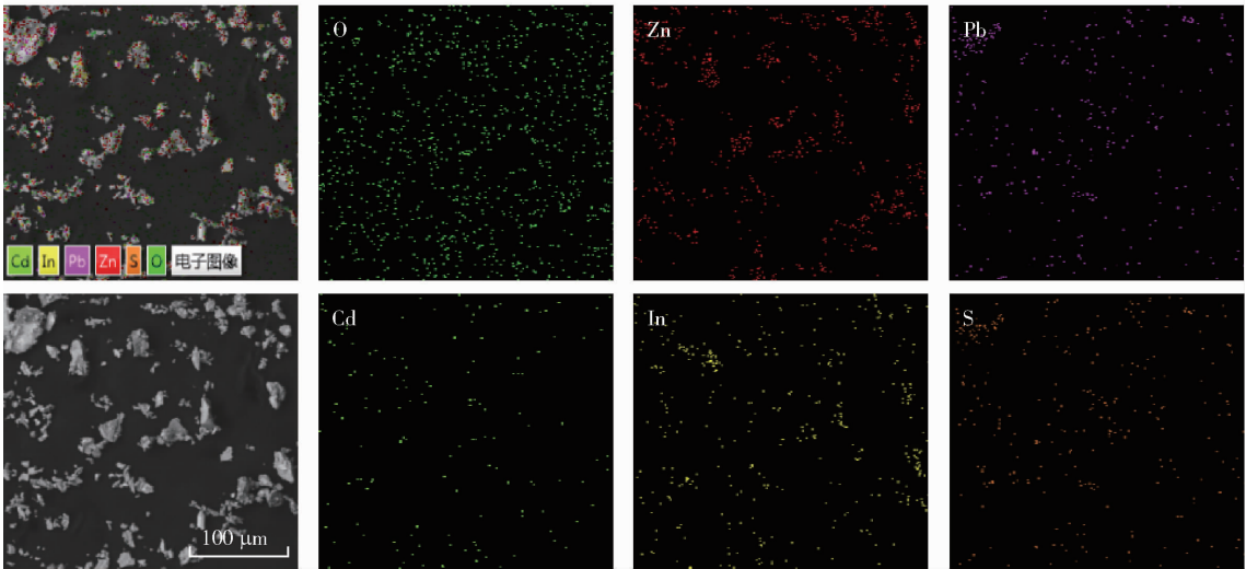
图 9 烟尘 SEM 图及 EDS 面扫描图
