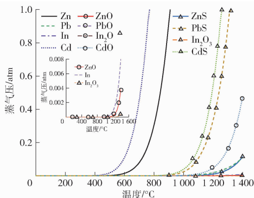
图4 饱和蒸气压与温度关系
