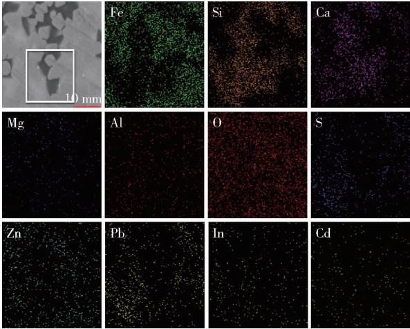
图 2 脱硫铅银渣的 SEM 图及 EDS 面扫描图 Fig. 2 SEM and EDS scanning of desulfurization lead-silver slag
