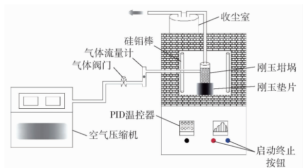
图3 试验设备连接示意
