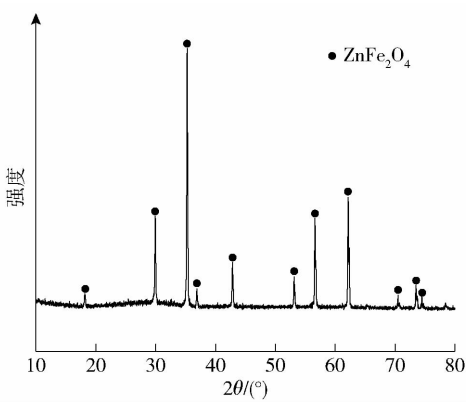
图 1 脱硫铅银渣的 XRD 图 Fig. 1 XRD of desulfurized lead-silver slag
