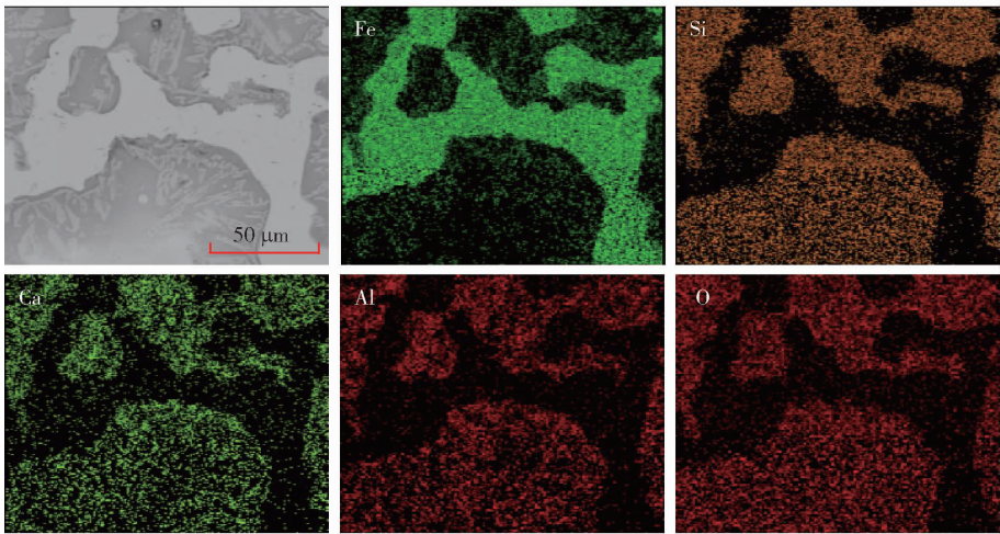
图 8 烟化渣 SEM 图及 EDS 面扫描图
