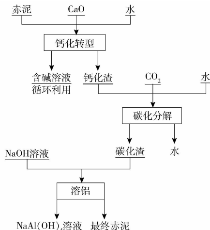
图 5 “钙化-碳化法”处理赤泥工艺流程
