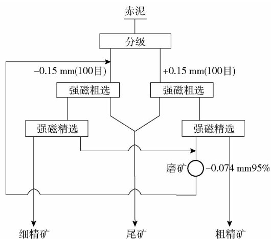
图 4 赤泥强磁选试验流程
