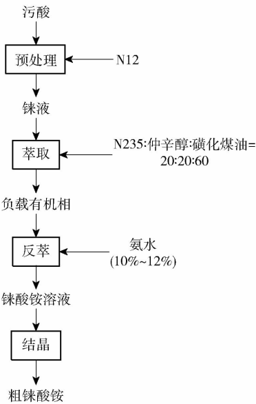
图 1 污酸中回收铼的新工艺路线
