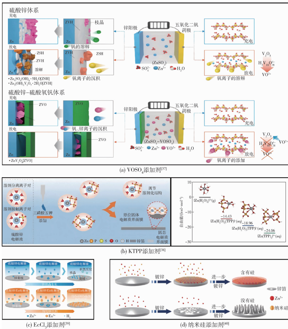
图3 \text{ZnSO}_4 电解液中(a) \text{VOSO}_4 添加剂 [37] , (b) KTPP 添加剂 [38] , (c) \text{EuCl}_3 添加剂 [39] 和(d) 纳米硅添加剂 [40] 的作用机理示意图
