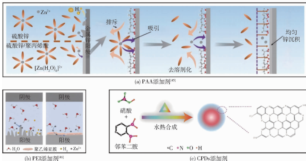
图5 \text{ZnSO}_4 电解液中(a) PAA 添加剂 [45] , (b) PEI 添加剂 [46] 的作用机理示意图和 (c) CPDs 添加剂 [47] 的设计思想
