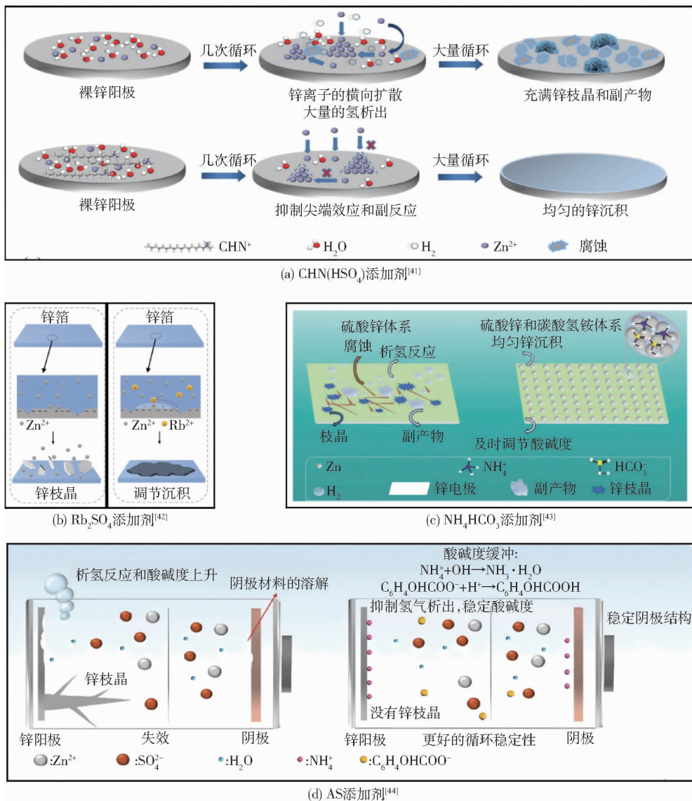
图4 \text{ZnSO}_4 电解液中(a) \text{CHN}(\text{HSO}_4) 添加剂 [41] , (b) \text{Rb}_2\text{SO}_4 添加剂 [42] , (c) \text{NH}_4\text{HCO}_3 添加剂 [43] 和(d) AS 添加剂 [44] 的作用机理示意图
