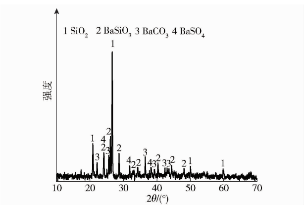
图 1 钡渣的 XRD 图谱
