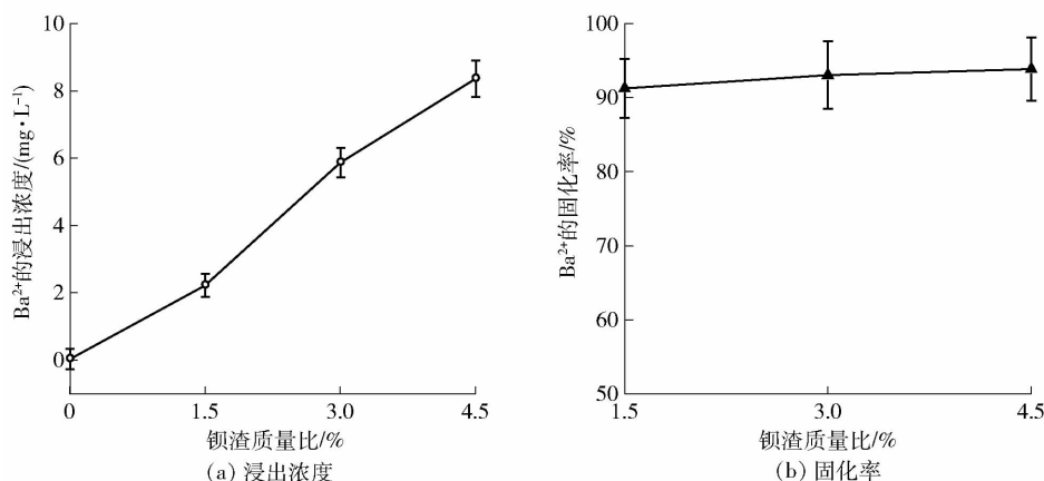
图8 不同胶砂试样 Ba^{2+} 浸出规律随钡渣添加量变化的曲线
