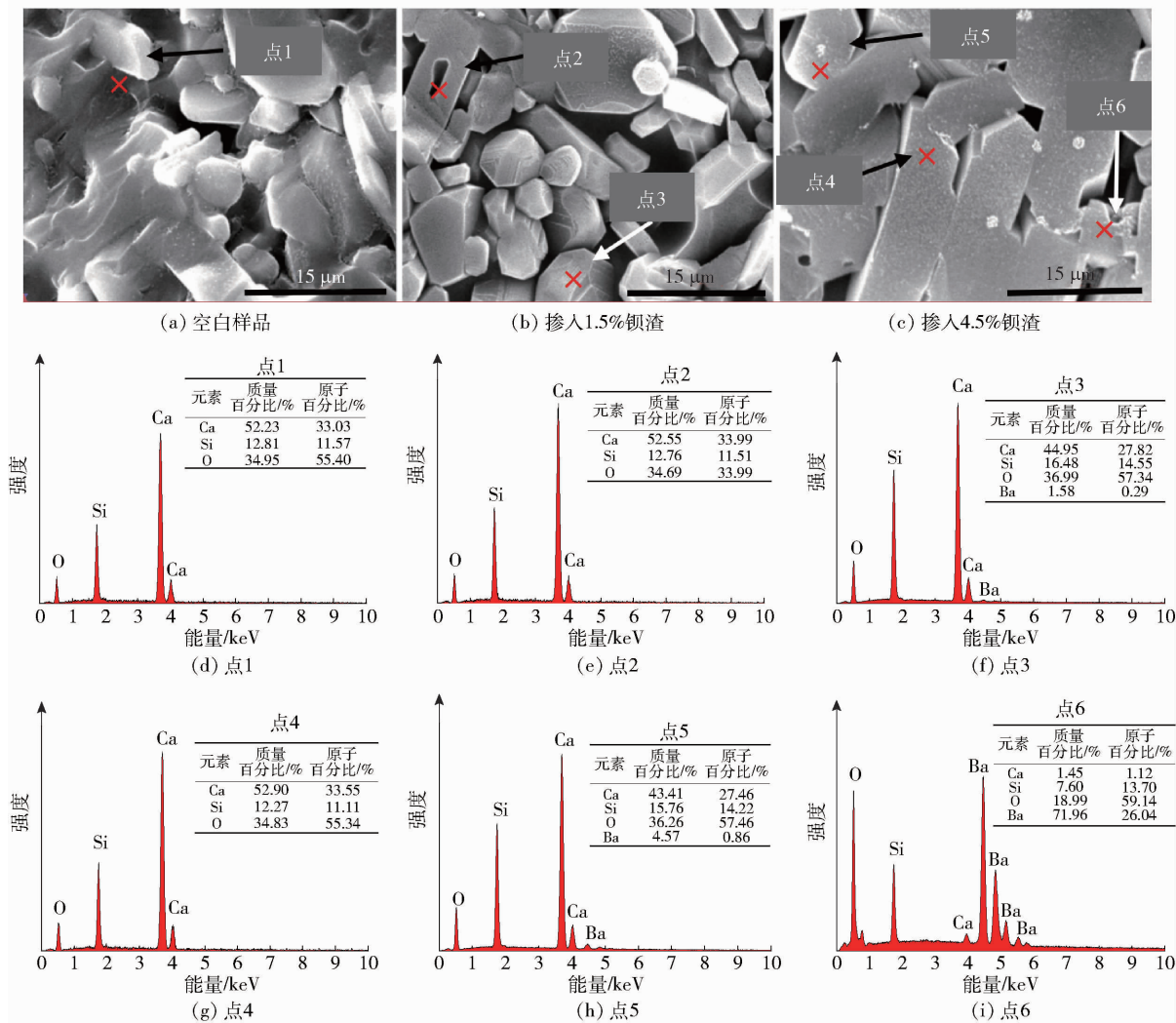
图 5 不同水泥熟料的 SEM 形貌图及 EDS 谱图
