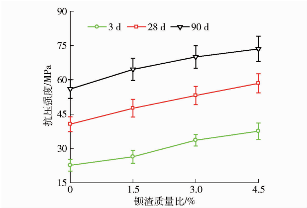
图 6 胶砂试样的抗压强度随钡渣添加量变化的曲线
