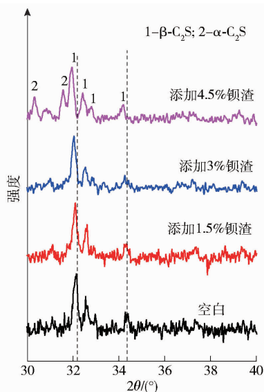
图 4 不同 \text{C}_2\text{S} 系列样品的 XRD 图谱
