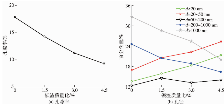
图7 胶砂试样的孔隙率和孔径随钡渣添加量变化的关系曲线
