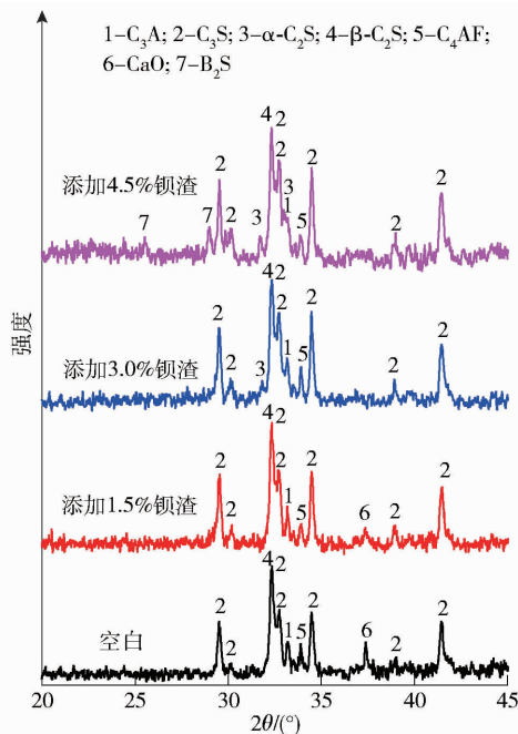
图 3 不同熟料样品的 XRD 图谱
