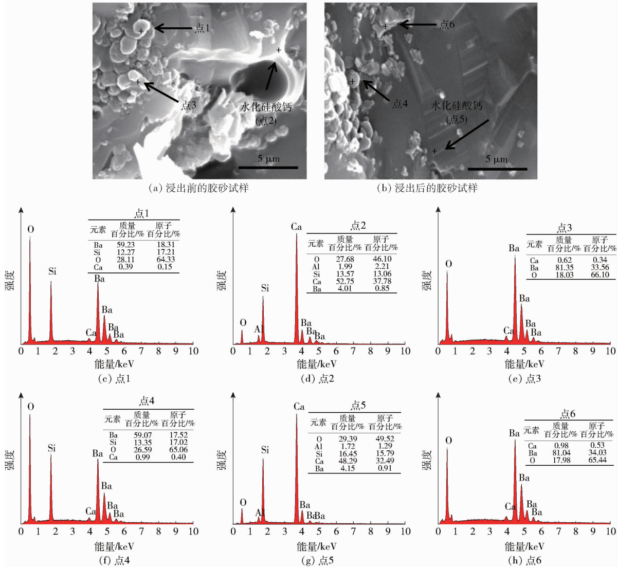
图9 浸出前后胶砂试样的 SEM 形貌图及 EDS 谱图
