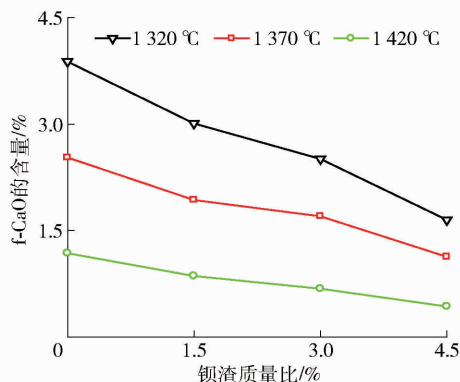
图 2 钡渣对水泥熟料中的 f-CaO 含量的影响曲线
