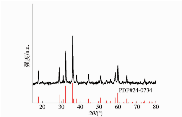
图 12 产品的 XRD 图 Fig. 12 The XRD pattern of the product
