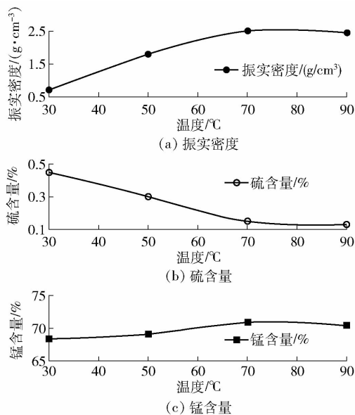
图 8 反应温度对四氧化三锰产品的影响
