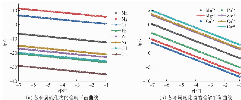
图4 金属元素的析出顺序
