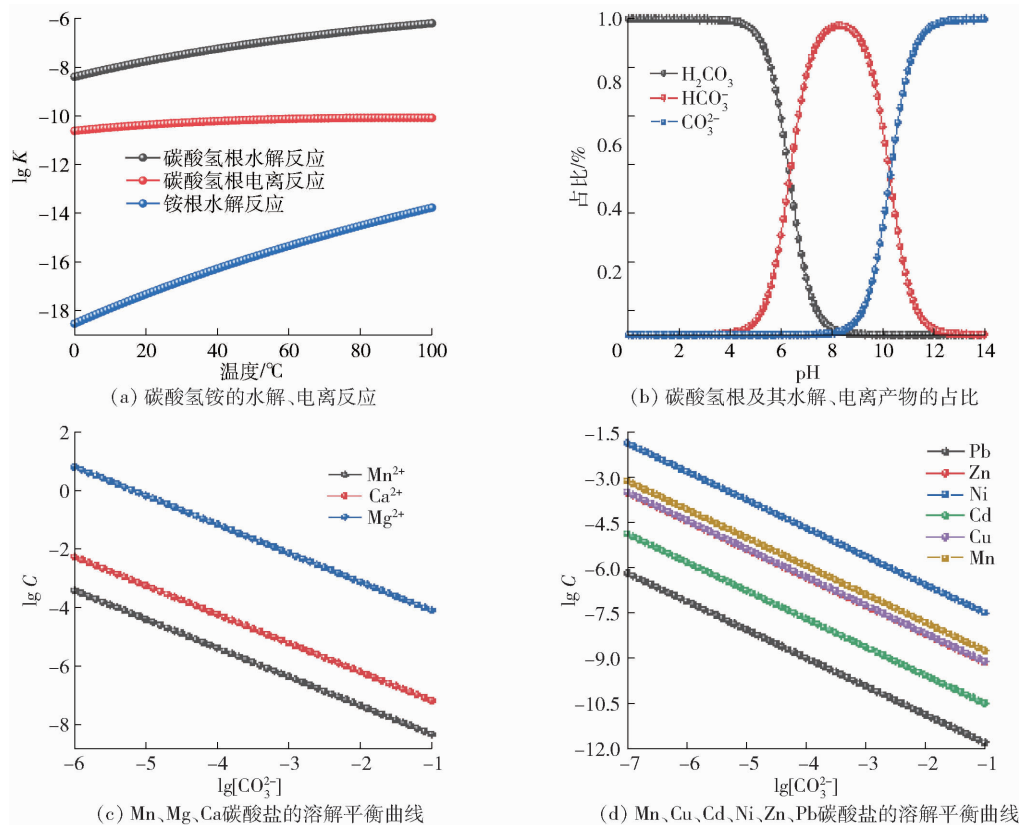
图 3 沉淀过程可能发生的相关反应
