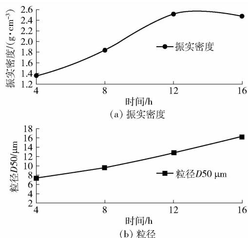
图9 反应时间对四氧化三锰产品的影响
