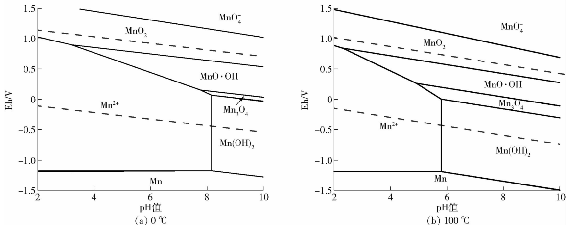
图5 不同温度下 Mn-H_2O 系的 Eh-pH 图
