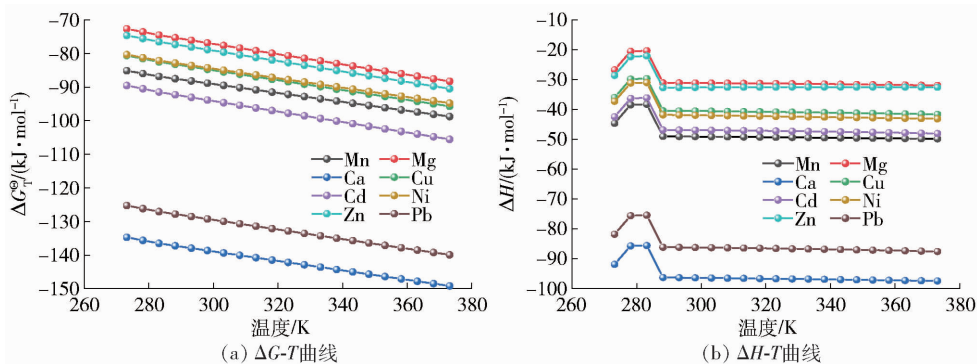
图2 浸出过程反应的 \Delta G 和 \Delta H 与温度的关系
