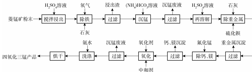
图1 菱锰矿酸浸液制备四氧化三锰流程图
