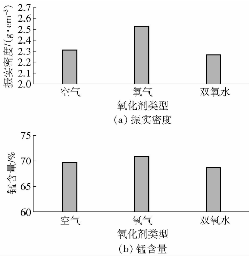
图 6 不同氧化剂对四氧化三锰产品的影响
