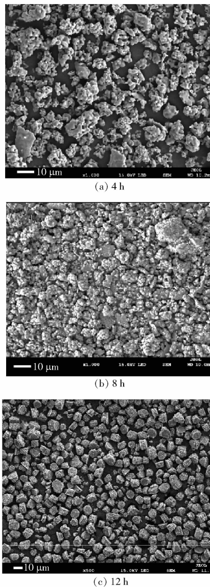
图10 不同反应时间条件下四氧化三锰产品的 SEM 图
