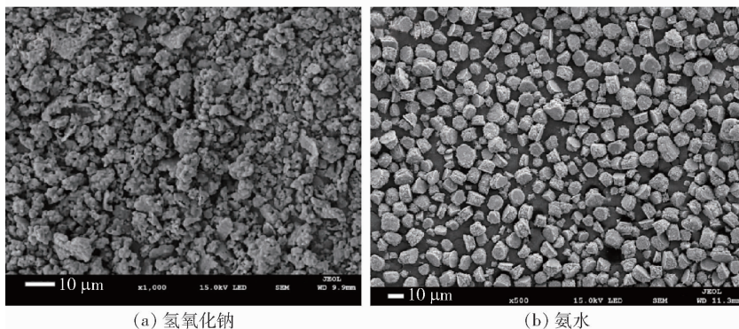
图 7 不同中和剂制备的四氧化三锰产品的 SEM 图
