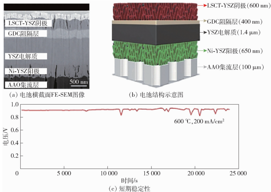
图2 Ni-YSZ 阳极支撑型电池结构及稳定性测试 [20]
