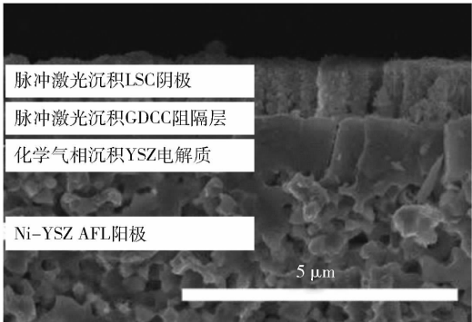
(a) 化学气相沉积法制备的YSZ电解质微观形貌图
