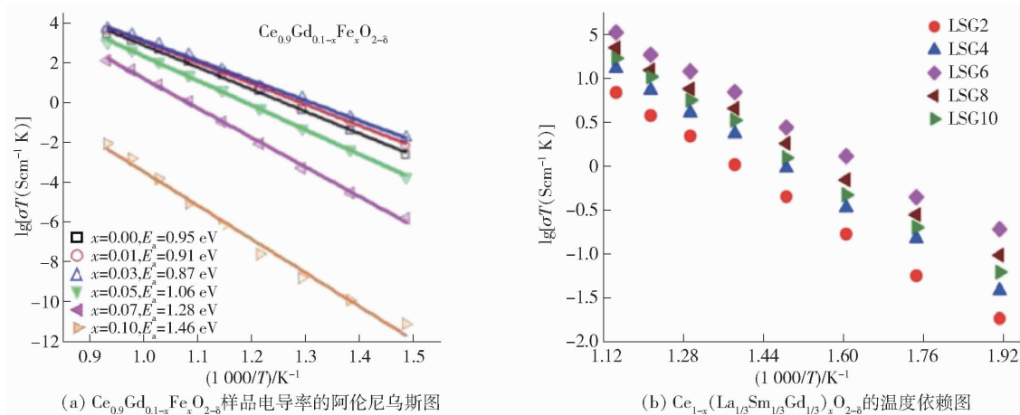
图4 掺杂 CeO 2 基电解质的离子电导率 [45, 46]
