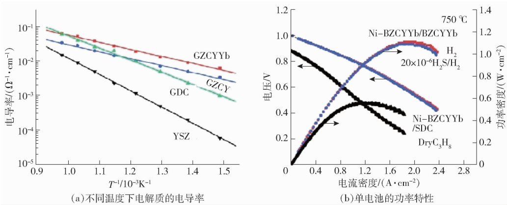
图 5 不同温度下电解质的电导率及对应单电池的功率特性 [56, 57]
