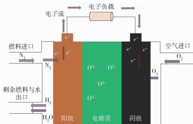
图 1 SOFC 的组成结构 [7]
