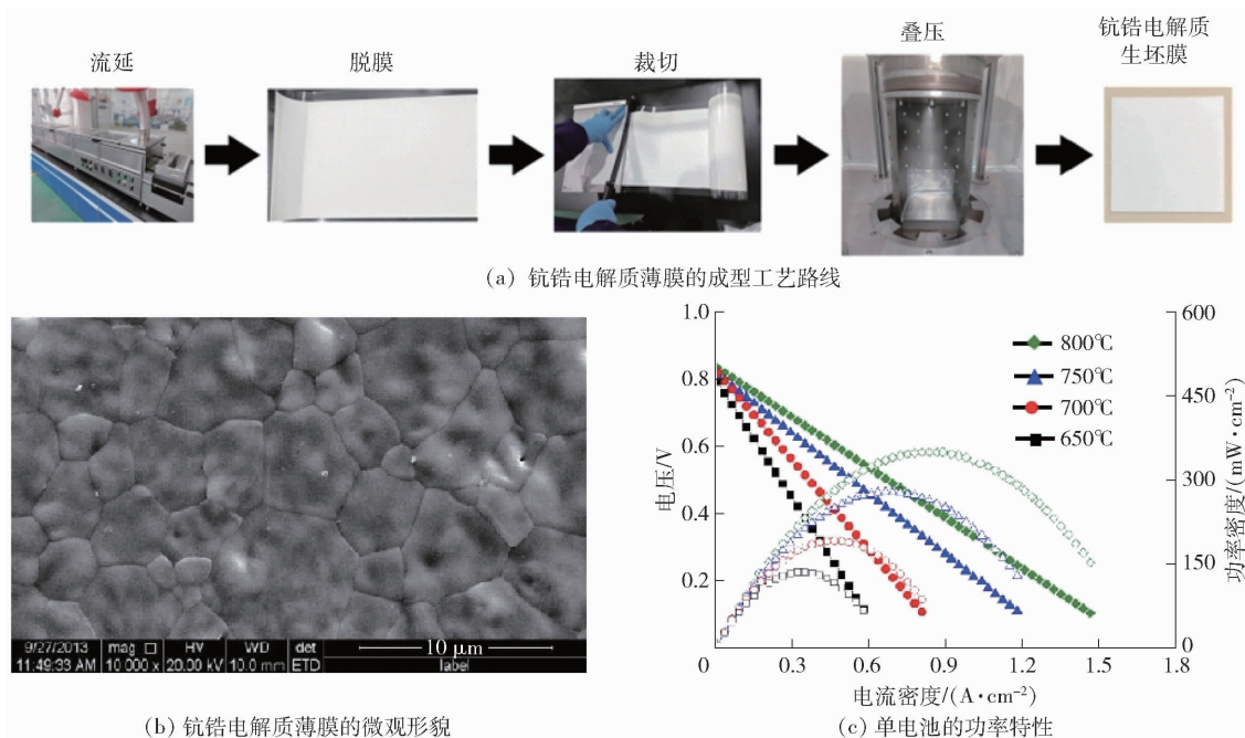
图 7 钪锆电解质薄膜的成型工艺路线及相关性能 [64]
