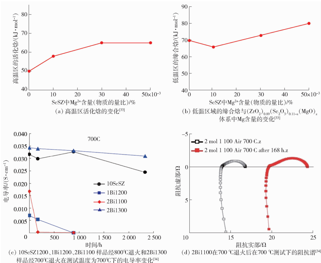
图3 共掺杂 ScSZ 电解质的电化学性能 [33, 34]
