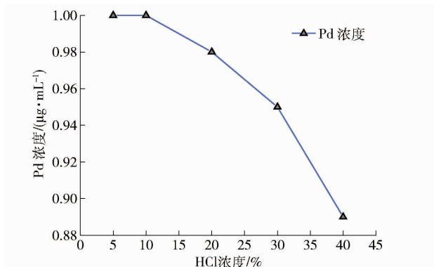
图4 HCl 浓度对钯测定的影响
