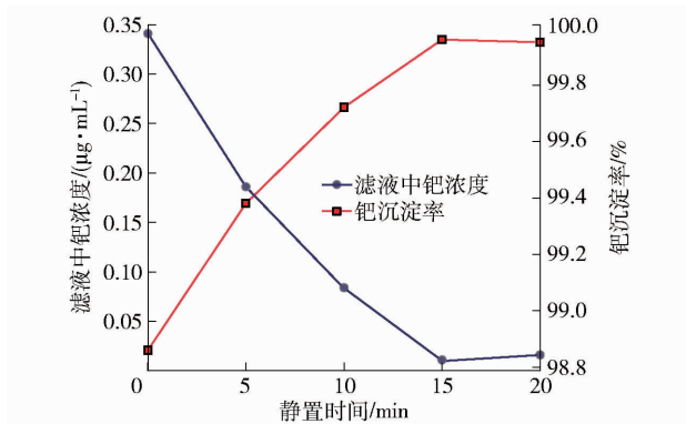
图3 静置时间对钯沉淀效果的影响
