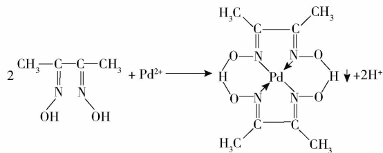
图 1 钯与丁二酮肟反应式
