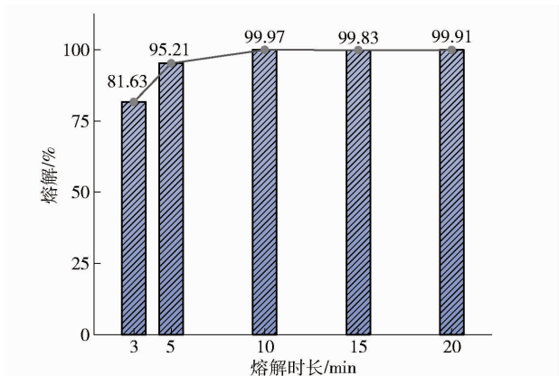
图2 熔融时间对试样熔解率的影响
