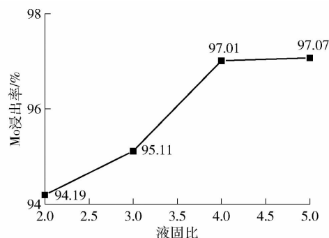
图 11 不同液固比下浸出结果
