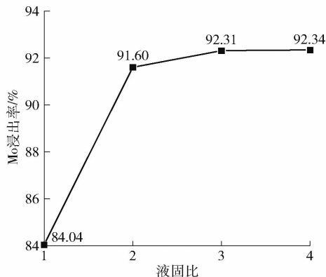
图 5 不同液固比下的浸出结果
