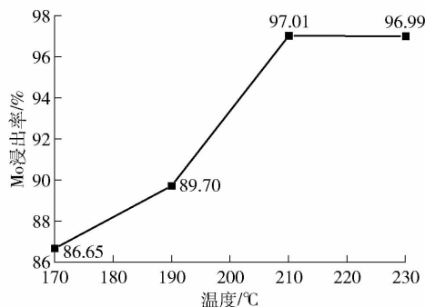
图 9 不同温度下浸出结果
