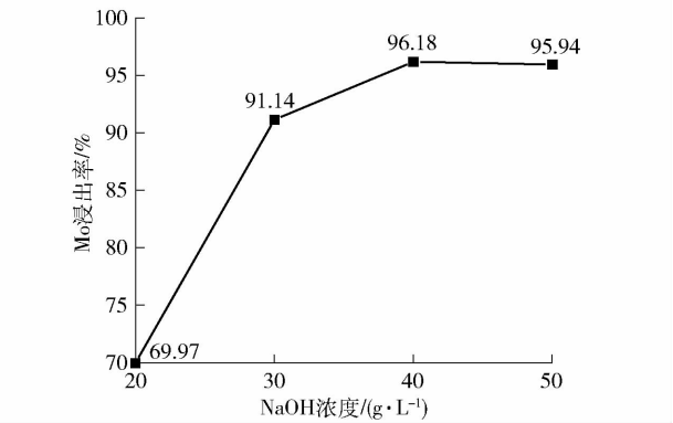
图 7 不同氢氧化钠用量下浸出结果 Fig. 7 Leaching results under different sodium hydroxide dosages
