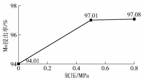
图 10 不同氧压下浸出结果
