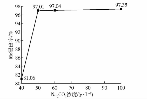
图 8 不同碳酸钠用量下浸出结果 Fig. 8 Leaching results under different sodium carbonate dosages
