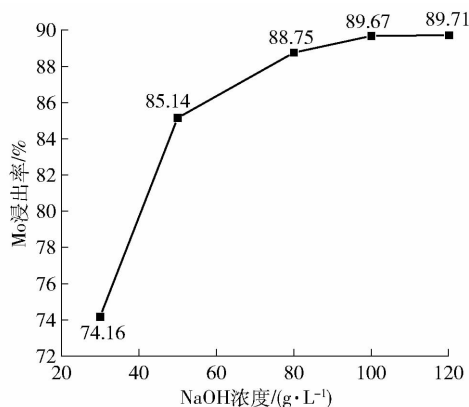
图 2 不同氢氧化钠用量下的浸出结果
