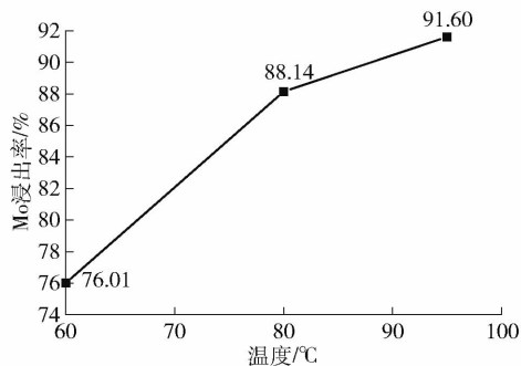
图 6 不同温度下的浸出结果
