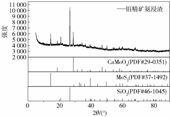
图 1 氨浸渣 XRD 分析
