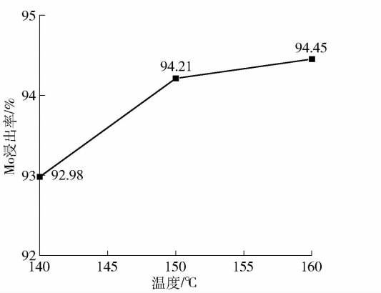
图 12 降成本优化浸出结果 Fig. 12 Cost-reducing optimization leaching results
