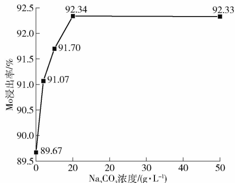
图 4 不同碳酸钠用量下的浸出结果
