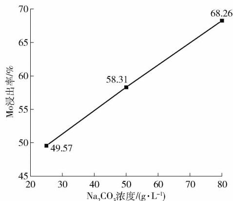
图 3 碳酸钠浸出结果
