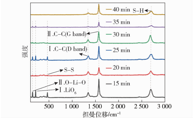
图 6 不同硫化温度下锂/石墨复合物的 Raman Fig. 6 Raman spectra of lithium/graphite composites at different sulfidation temperatures
