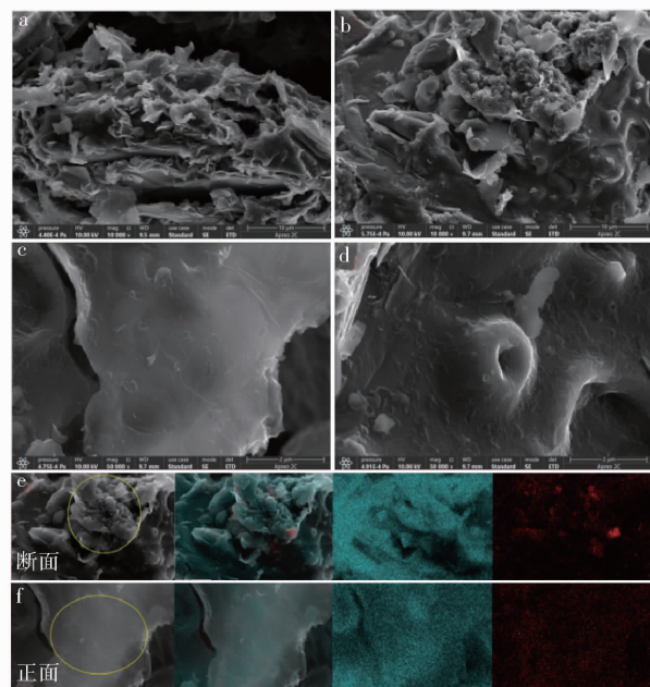
(a~d) - 粉末状锂/石墨复合物不同位置的高倍电镜; (e~f) - 粉末状锂/石墨复合物的断面和正面 EDS 面扫
