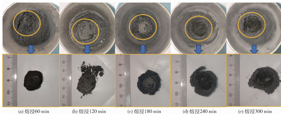
图2 不同熔浸时间下锂浸入石墨层实物图
