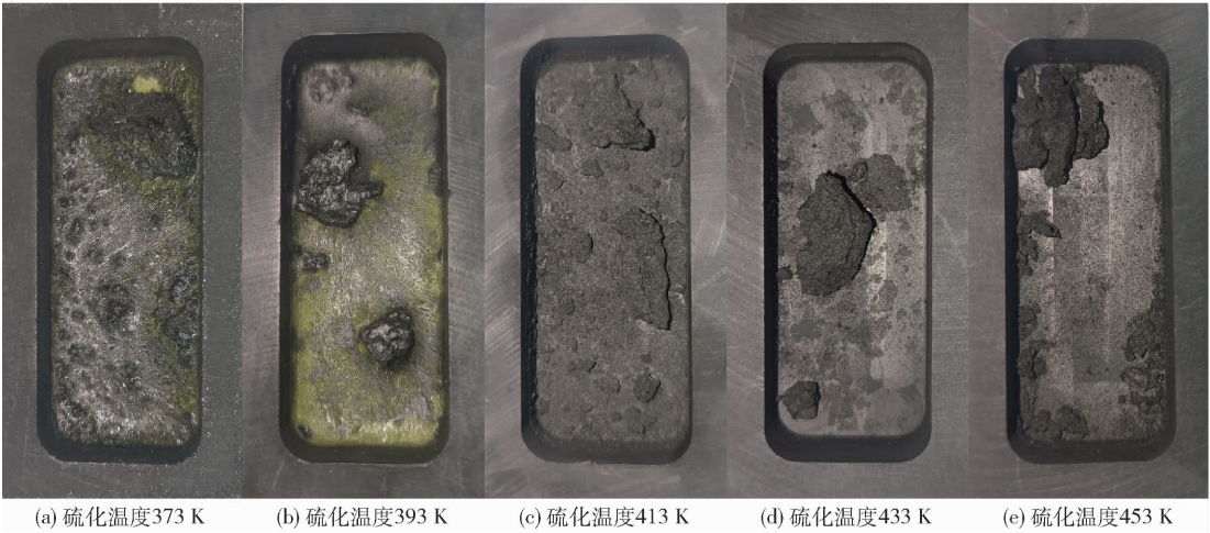
图 3 不同硫化温度下锂/石墨复合物硫化实物图
