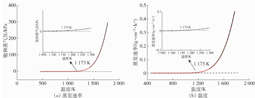
图 1 金属锂饱和蒸气压和蒸发速率与温度的关系
