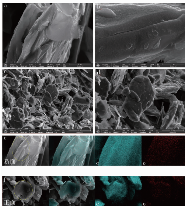
(a~d) - 块状锂/石墨复合物不同位置的高倍电镜; (e~f) - 块状锂/石墨复合物的断面和正面 EDS 面扫
