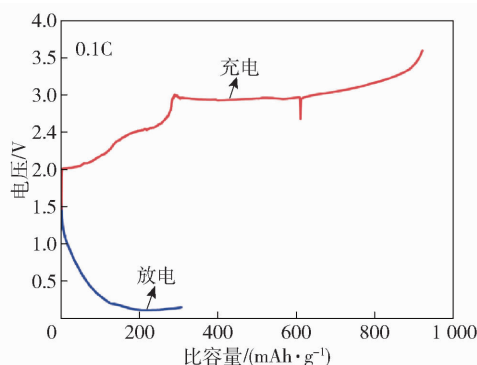
图 10 硫化锂/石墨复合材料正极的首圈比容量(0.1 C)
