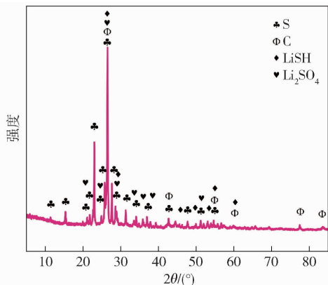
图 9 硫化锂/石墨复合物的 XRD
