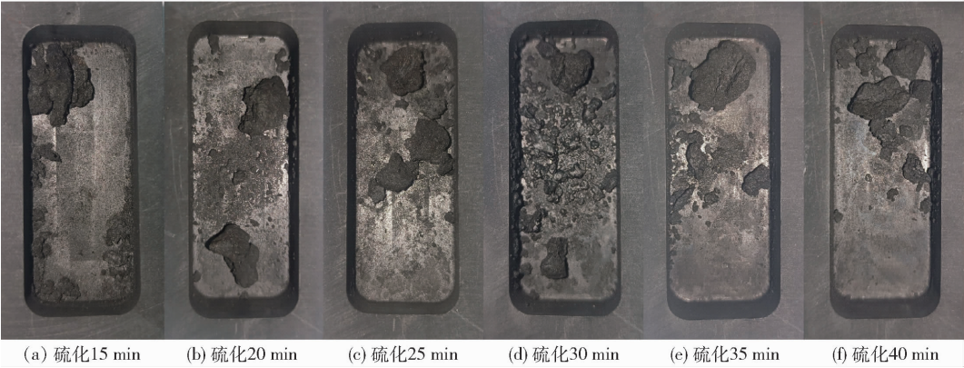
图 5 不同硫化时间下锂/石墨复合物硫化实物图
