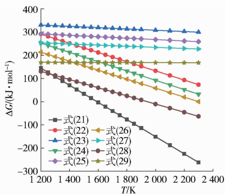
图 5 碳热还原其他氧化物的 \Delta G_r^\theta - T 图
