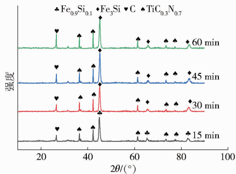
图 17 不同还原时间下对应的 x 射线衍射图谱
