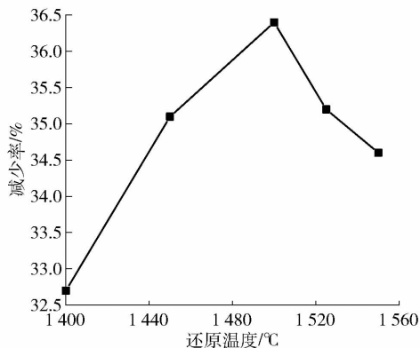
图 11 还原温度对还原后样品质量的影响
