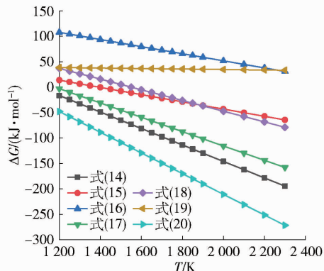
图4 CO 还原 \text{FeTiO}_3 的 \Delta G_r^\theta - T 图
