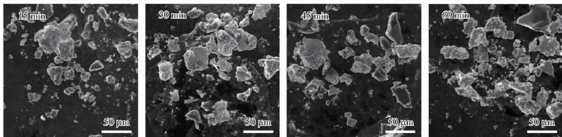
图 19 不同还原时间下还原产物局部微观形貌图(1 000 ×)
