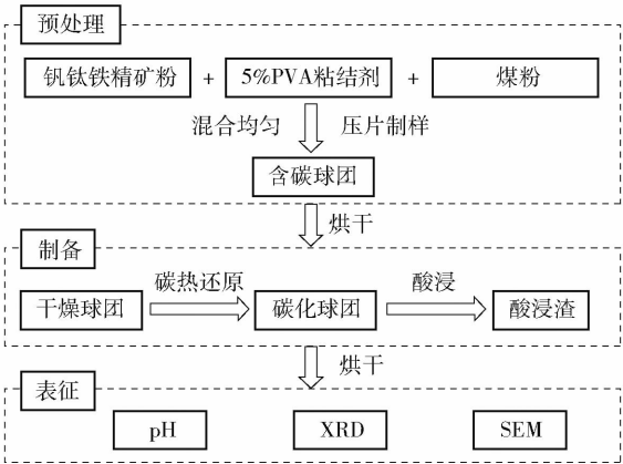
图 1 工艺流程图
