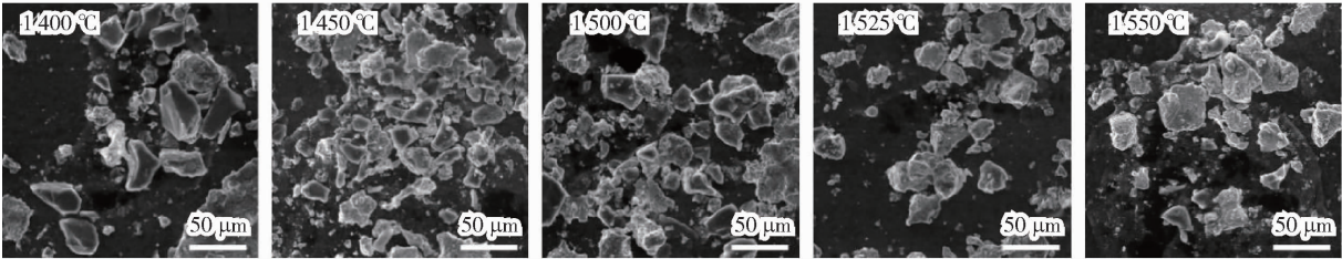
图 14 不同还原温度下还原产物局部微观形貌图(1 000 ×)
