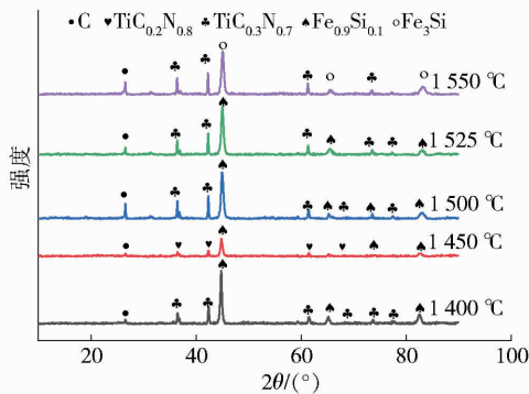
图 12 不同还原温度下对应 X 射线衍射图谱
