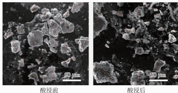
图 22 酸浸前后产物局部微观图
