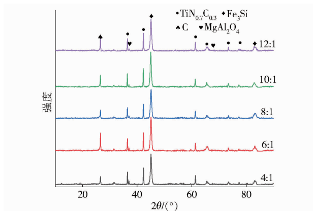
图7 不同球料比下还原产物X射线衍射图谱
