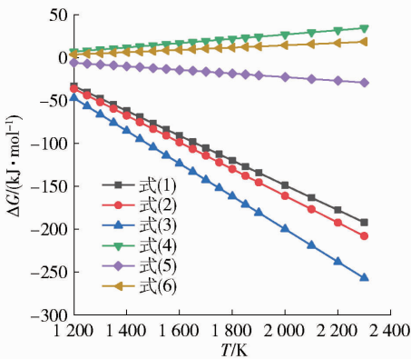
图 2 碳热还原铁氧化物的 \Delta G_r^{\theta} - T 图
