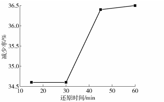
图 16 不同还原时间下质量变化趋势
