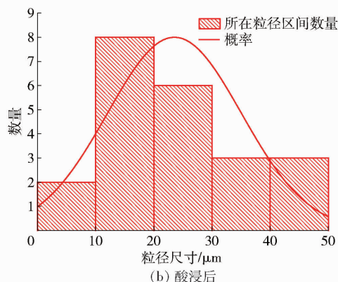
图 23 酸浸前后粒径尺寸分布
