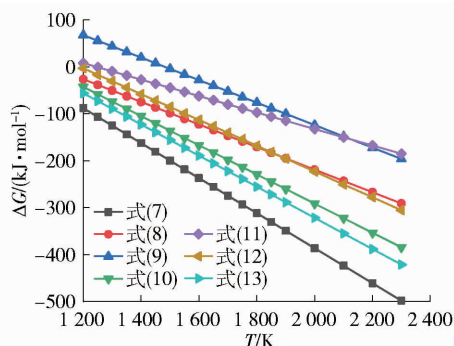
图3 C 还原 \text{FeTiO}_3 的 \Delta G_r^\theta - T 图
