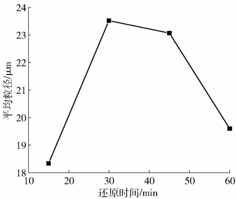
图 20 不同还原时间下还原产物平均粒径变化趋势
