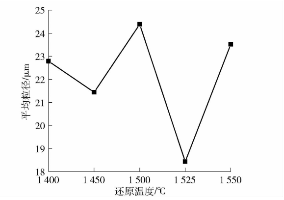
图 15 不同还原温度下还原产物平均粒径变化趋势
