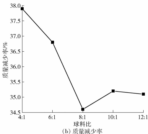
图6 球料比对物料中位粒径和还原后产物质量的影响
