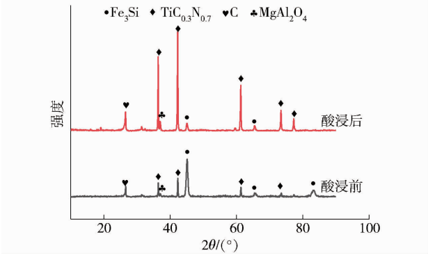
图 21 酸浸前后 X 射线衍射图谱
