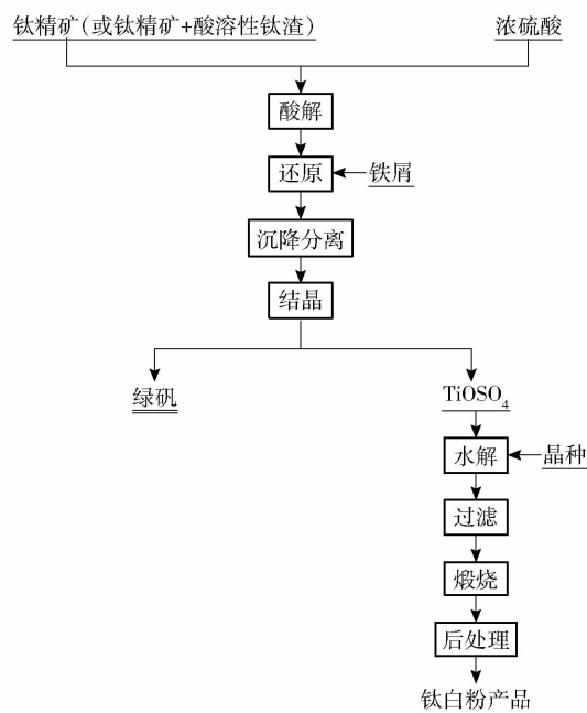
图 1 硫酸法钛白工艺流程
