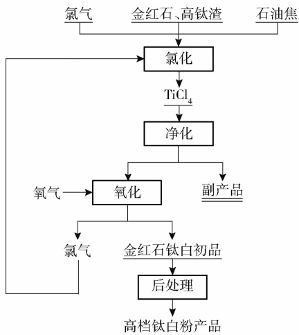
图2 氯化法钛白生产工艺流程
