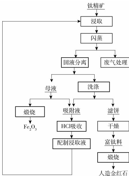
图3 盐酸法钛白粉生产工艺流程
