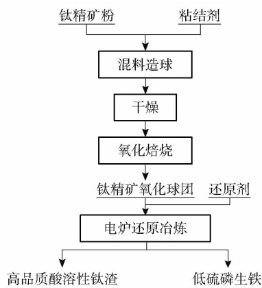
图 7 电炉冶炼高品质酸溶性钛渣工艺流程
