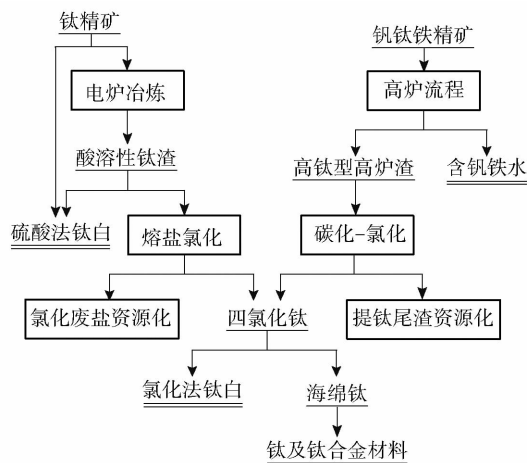
图4 四川省攀西地区钛冶炼工艺
