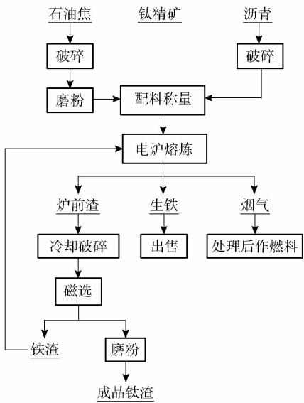
图 6 攀钢钛渣冶炼工艺流程
