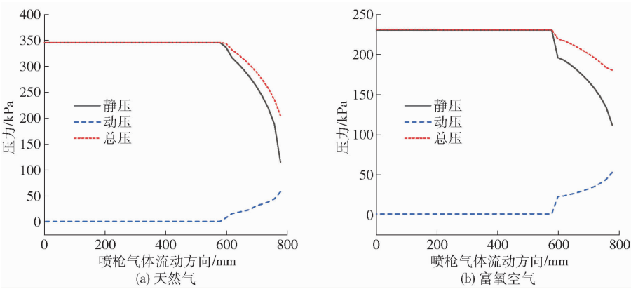
图 10 不同孔道截面平均压力沿喷枪流动方向变化趋势
