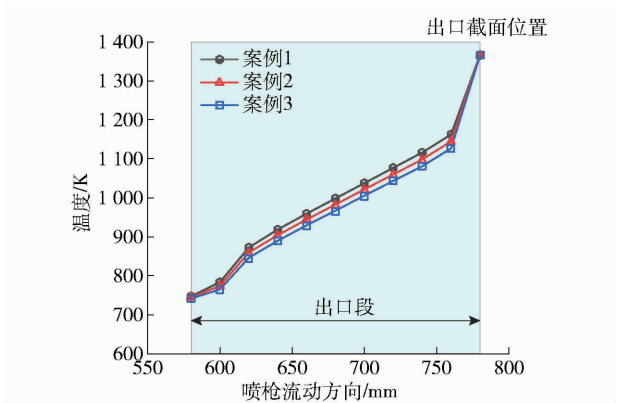
图 13 不同流量下喷枪截面平均温度随流动方向的变化趋势
