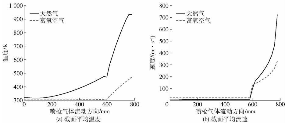
图 7 天然气及富氧空气沿喷枪流动方向不同物理量的变化趋势
