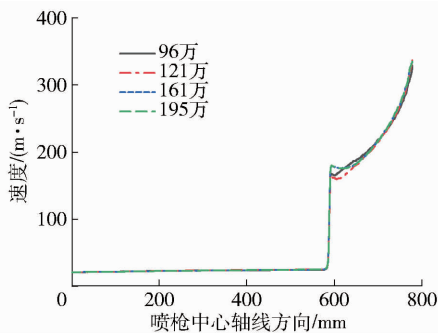
图3 不同网格数下喷枪中心轴线沿喷吹方向速度变化趋势
