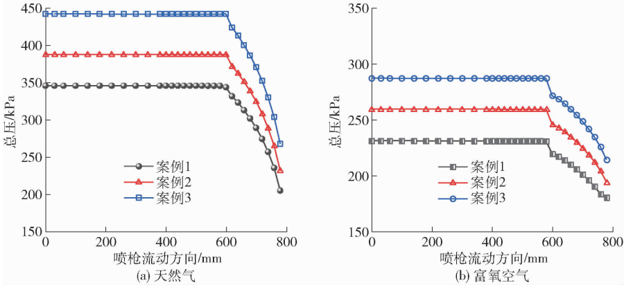
图 11 不同流量下孔道截面平均总压沿喷枪流动方向变化趋势
