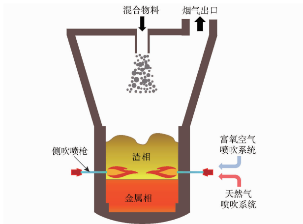
图1 阳极泥侧吹炉冶炼示意图
