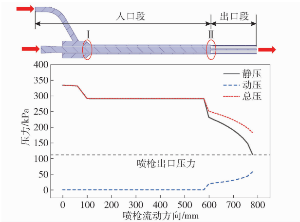
图 9 喷枪气流孔道截面平均压力随流动方向变化趋势
