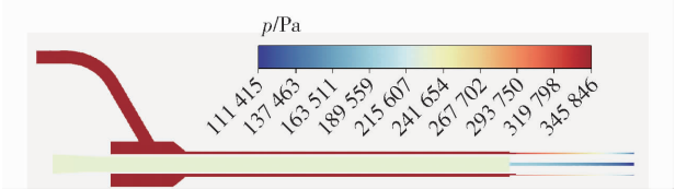
图 8 喷枪中心截面压力分布
