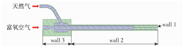
图 5 喷枪流动方向截面示意图 Fig. 5 Cross-section of the flow direction of the lance
