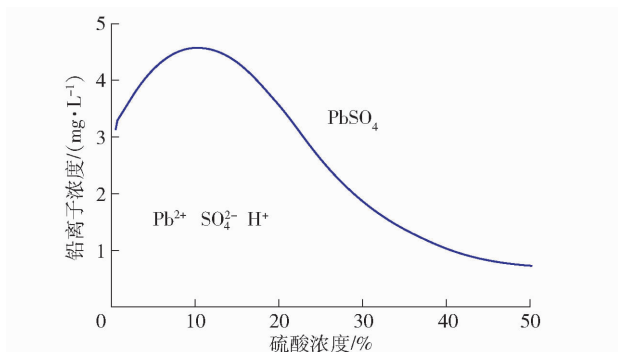
图 1 硫酸铅在硫酸中的溶解度曲线 [11]
