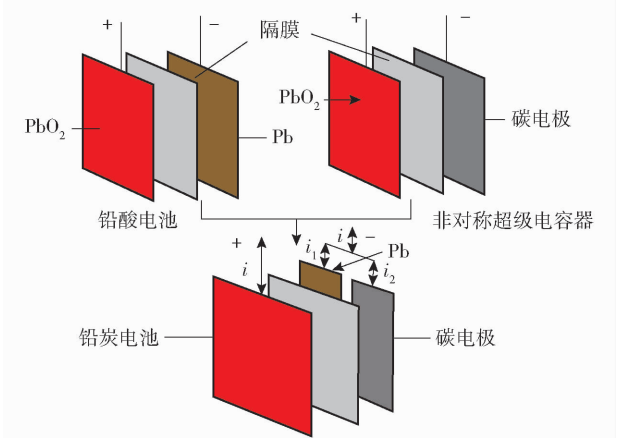
图 3 铅炭电池配置示意图 [15]
