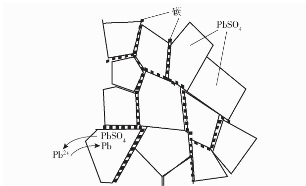
图 2 碳材料加入负极后形成的导电网络 [13]
