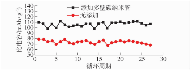
图 4 添加 MWCNT 与不添加 MWCNT 的测试 电池循环寿命数据对比 [20]
