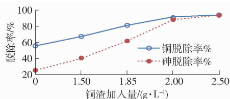
图 2 铁粉过量系数 1.5 倍条件下铜渣加入量对铜、砷去除率的影响
