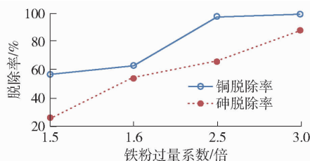
图 1 不加入铜渣条件下铁粉过量系数对铜、砷去除率的影响
