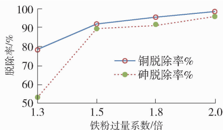
图3 铜渣加入量 2.00 g/L 条件下铁粉过量系数对铜、砷去除率的影响
