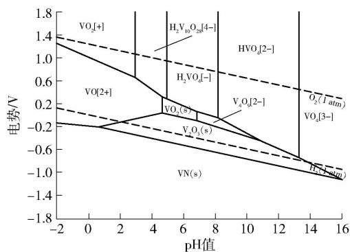
图 3 V-N-O-H 系 E -pH 图
