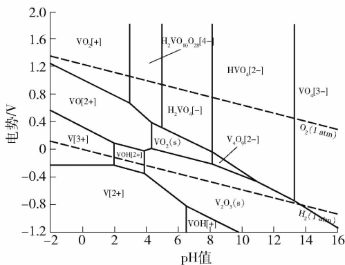
图 2 V-O-H 系 E -pH 图
