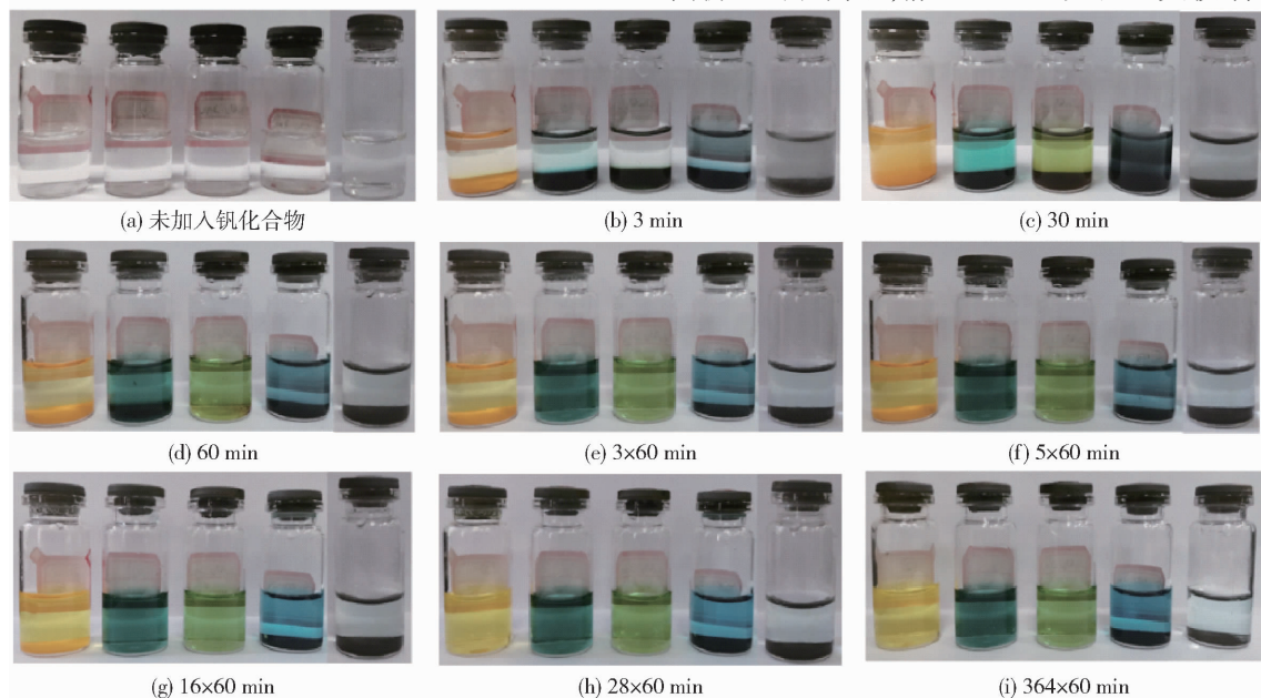
图 4 不同浸泡时间下钒化合物的溶解照片(从左到右依次为 V_2O_5 、 NaV_2O_5 、 VO_2 、 V_2O_3 、VN)
