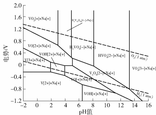
图 1 V-Na-O-H 系 E -pH 图
