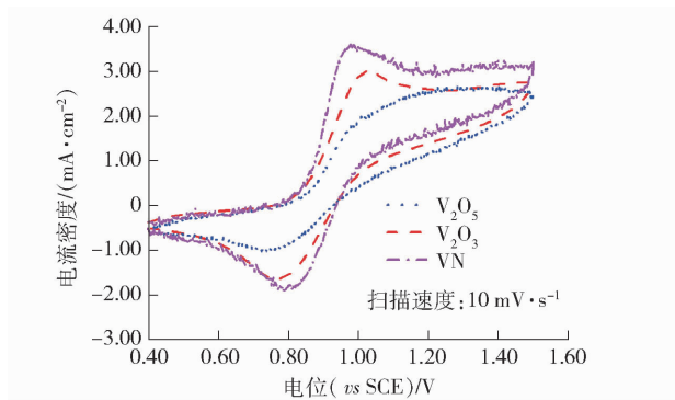
图 8 \text{V}_2\text{O}_5 、 \text{V}_2\text{O}_3 、VN 在 0.1 \text{ mol} \cdot \text{L}^{-1} \text{V}^{4+} + 2.0 \text{ mol} \cdot \text{L}^{-1} \text{H}_2\text{SO}_4 中的循环伏安曲线
