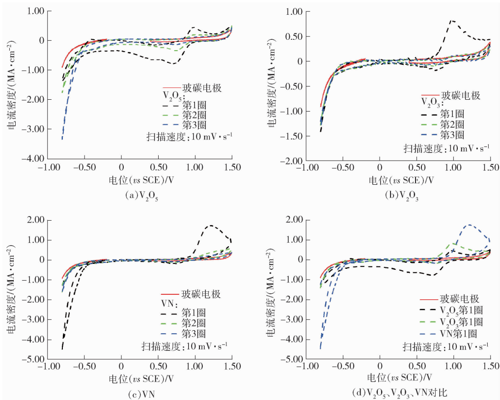
图6 3种钒化合物在 2.0 \text{ mol} \cdot \text{L}^{-1} \text{H}_2\text{SO}_4 中的循环伏安曲线
