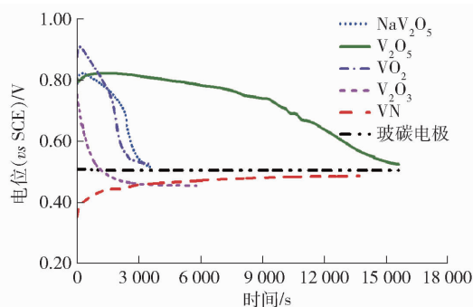
图 5 不同钒化合物在 1.5 \text{ mol} \cdot \text{L}^{-1} \text{VOSO}_4 + 2.0 \text{ mol} \cdot \text{L}^{-1} \text{H}_2\text{SO}_4 电解液中的开路电位
