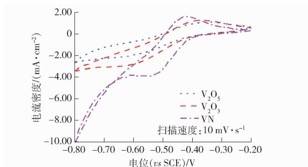
图 7 \text{V}_2\text{O}_5 、 \text{V}_2\text{O}_3 、VN 在 0.1 \text{ mol} \cdot \text{L}^{-1} \text{V}^{3+} + 2.0 \text{ mol} \cdot \text{L}^{-1} \text{H}_2\text{SO}_4 中的循环伏安曲线
