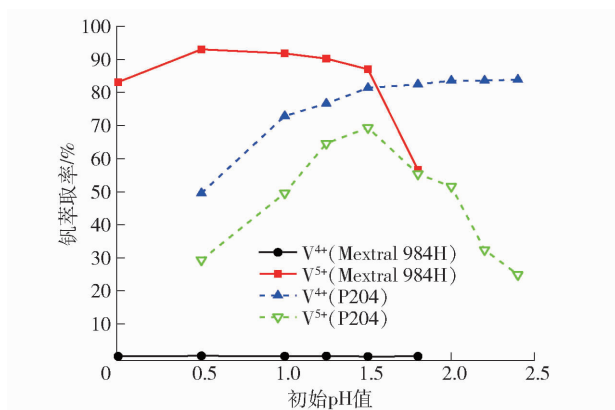
图 1 pH 值对钒萃取率的影响
