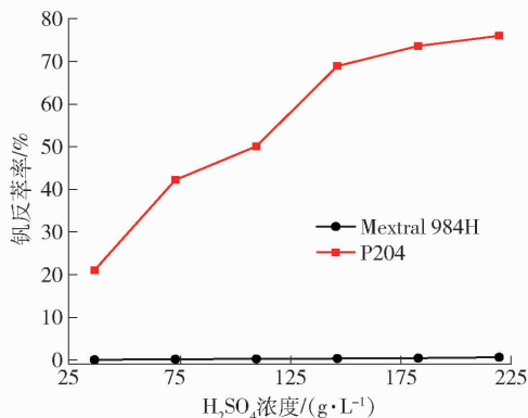
图 5 硫酸浓度对钒反萃率的影响
