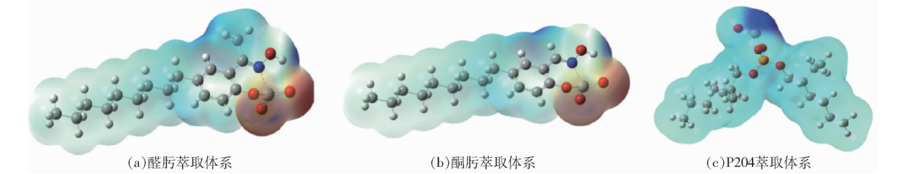
图2 钒萃合物的静电势
