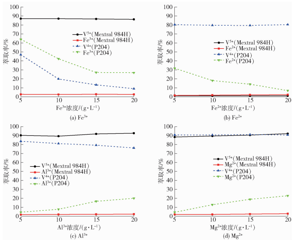
图 3 不同金属离子浓度对萃取率的影响
