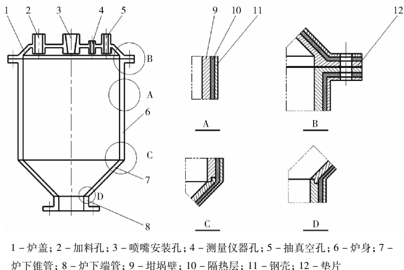
图 3 反应炉结构示意图
