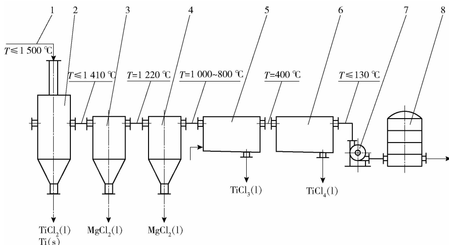
1 - 反应炉抽出炉气; 2 - 气液分离器; 3 - 冷却器 I; 4 - 冷却器 II; 5 - 冷凝器 I; 6 - 冷凝器 II; 7 - 抽风机; 8 - 氩气柜
