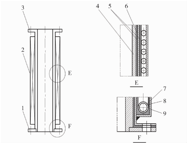
1 - 炉下端管；2 - 炉身感应线圈；3 - 炉上端管；4 - 坩埚壁；5 - 隔热层；6 - 内壳；7 - 铜管；8 - 隔离层；9 - 外壳。
