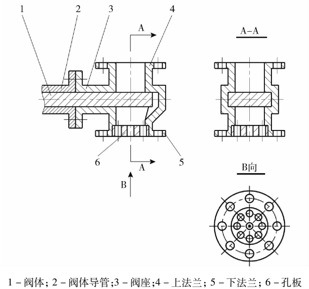
图 7 阀门(阀门 1、阀门 2)结构示意图
