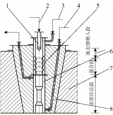
1 - 喷头；2 - 液态镁管；3 - 四氯化钛管；4 - 冷却水管；5 - 四氯化钛夹层管多孔段；6 - 冷却水夹层管；7 - 反应炉盖；8 - 隔热层
