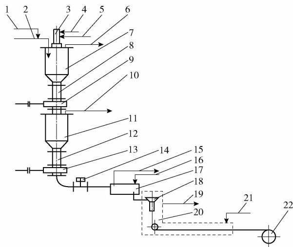
1 - 氩气管; 2 - 合金料管; 3 - 喷嘴; 4 - 液镁管; 5 - 四氯化钛管; 6 - 反应炉气抽出管; 7 - 反应炉; 8 - 中频感应炉; 9 - 阀门 1; 10 - 精炼炉气抽出管; 11 - 精炼炉; 12 - 高频感应炉; 13 - 阀门 2; 14 - 电磁流量计; 15 - 氩气抽出管; 16 - 氩气输入管; 17 - 连铸分配槽; 18 - 结晶器; 19 - 氩气抽出管; 20 - 密封仓; 21 - 氩气输入管; 22 - 钛材产品
