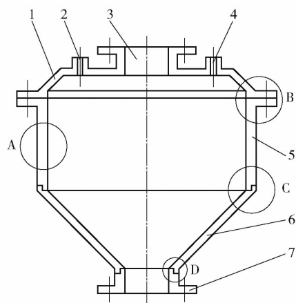
1 - 炉盖；2 - 测量仪器孔；3 - 炉上端管；4 - 抽真空孔；5 - 炉身；6 - 炉下锥筒；7 - 炉下端管；A、B、C、D 放大图见图 3。
