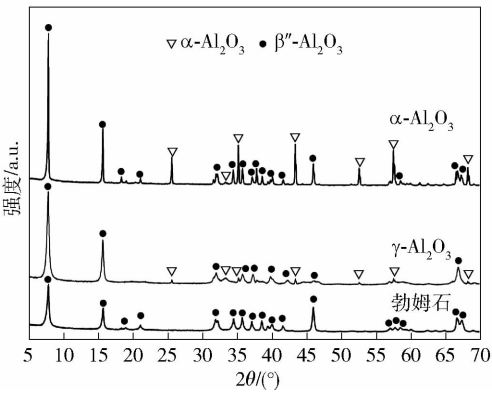
图 2 不同前驱体制备的 \beta'' - \text{Al}_2\text{O}_3 XRD 图谱
