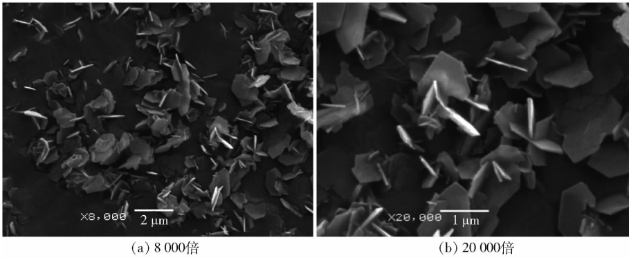
图 1 水热法制备的六边片状结构勃姆石 SEM 图
