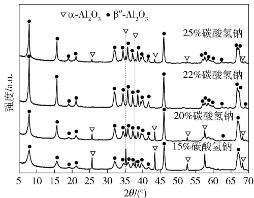
图4 不同加入量的碳酸氢钠制备 \beta'' - \text{Al}_2\text{O}_3 的 XRD 图谱
