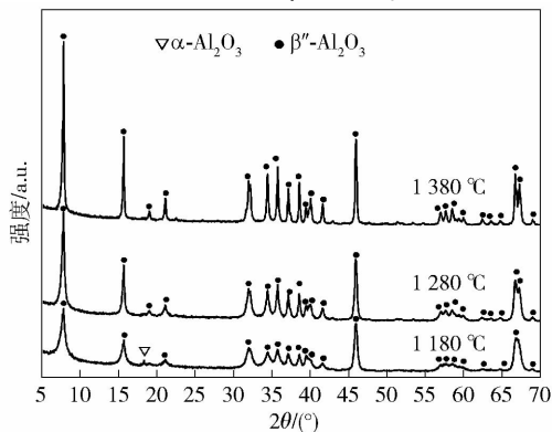
图5 不同温度煅烧后制备 \beta'' - \text{Al}_2\text{O}_3 的 XRD 图谱
