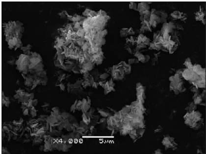
(c) 铝源为勃姆石
