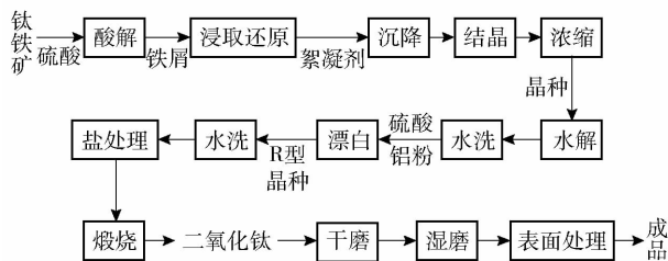
图1 硫酸法制备钛白工艺流程
