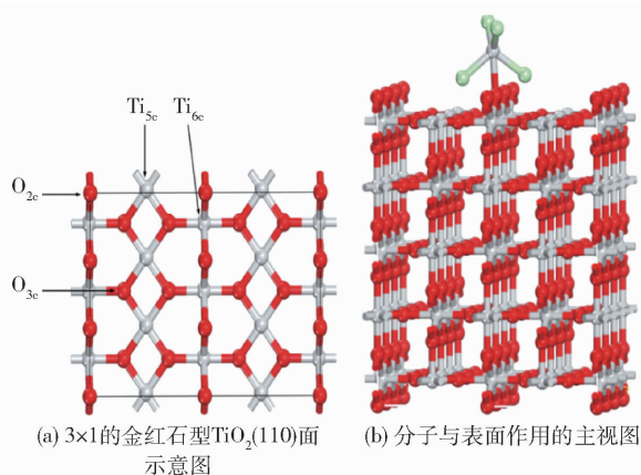
图 3 3 × 1 的金红石型 TiO 2 (110) 面示意图及分子与表面作用主视图
