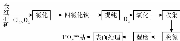
图 2 氯化法制备钛白工艺流程
