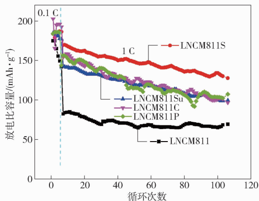
图 4 样品的循环曲线
