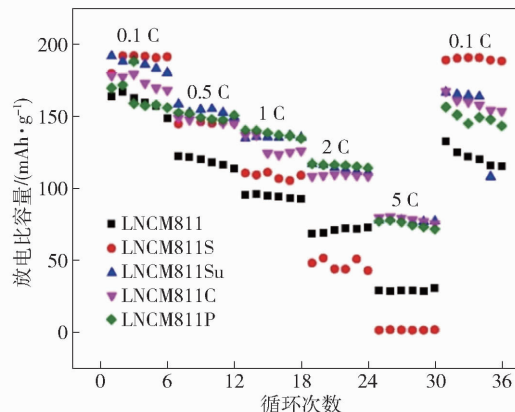
图 5 样品的倍率性能曲线
