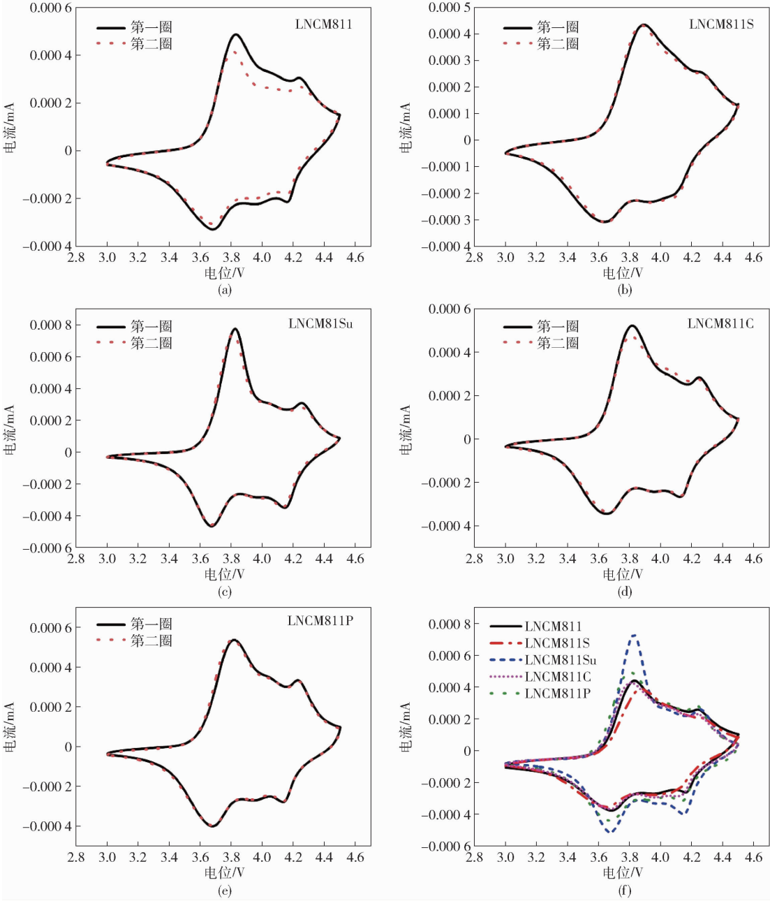
图 6 样品的循环伏安曲线(a-e)和第二圈的 CV 曲线(f)
