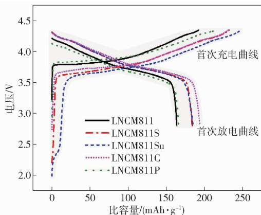
图 3 样品的首次充放电曲线
