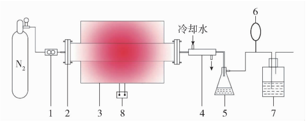
1-流量计;2-密封法兰;3-管式热解炉炉体;4-冷却管;5-收油瓶;6-气袋;7-碱液吸收瓶;8-电表
