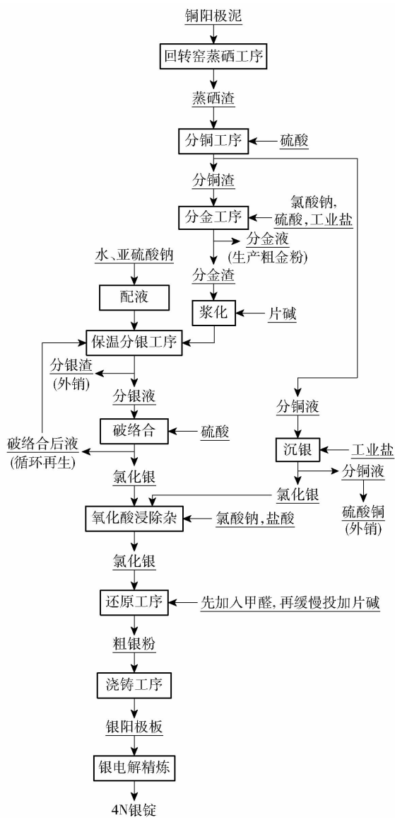
图4 亚钠分银-甲醛间接还原工艺流程
