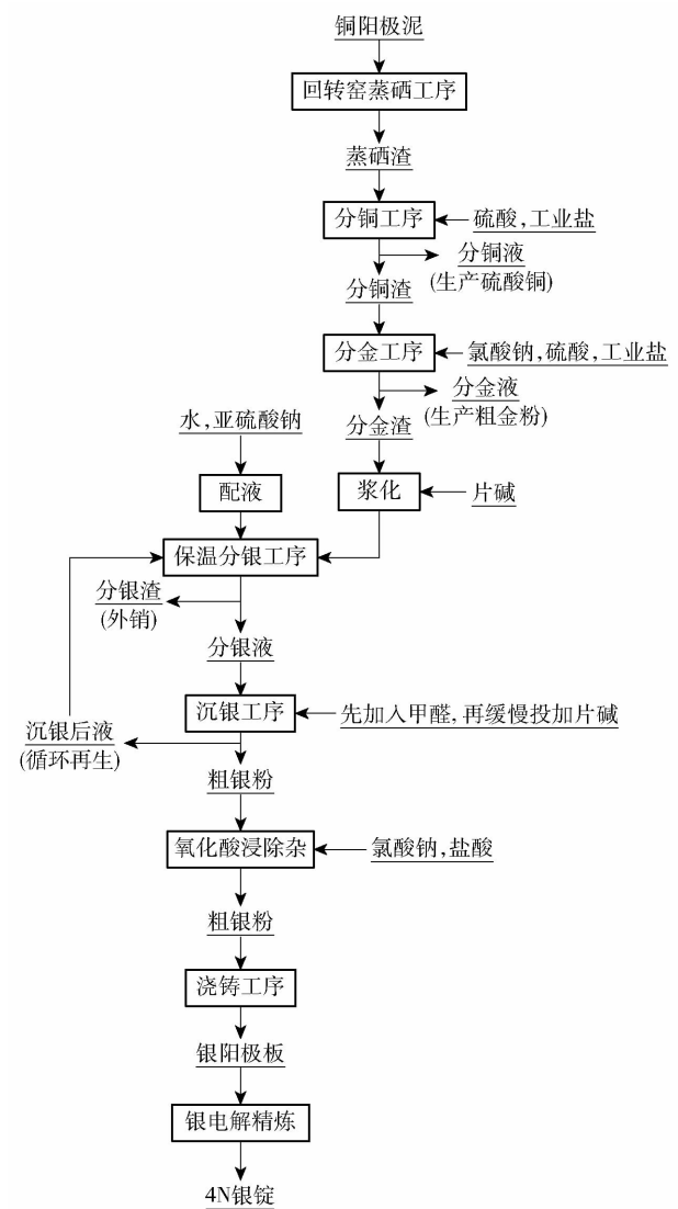
图3 亚钠分银-甲醛直接还原工艺流程
