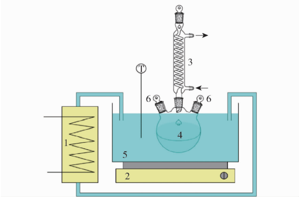
1 - 温度加热系统; 2 - 磁力搅拌装置; 3 - 冷凝管; 4 - 三孔圆底烧瓶; 5 - 水浴槽; 6 - 温度计
