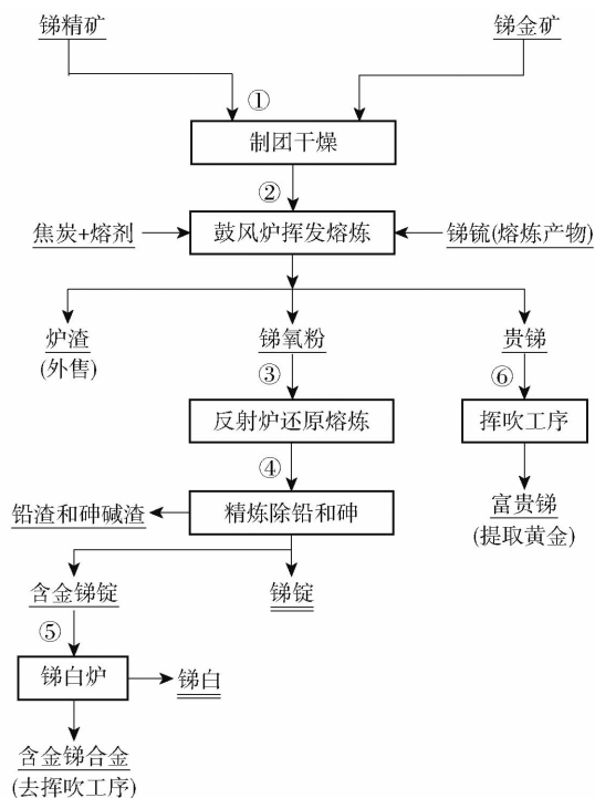
图1 锡精矿与锡金矿火法炼锡工艺示意
