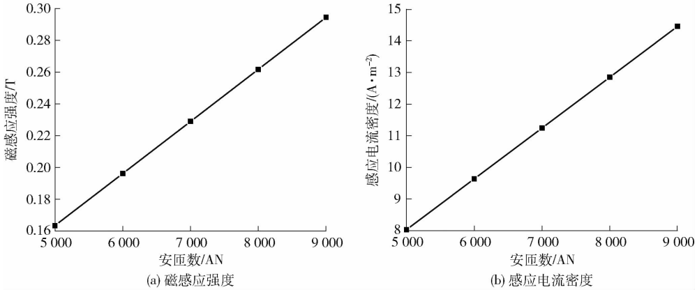
图 9 底部线圈正弦波电流 6 000 ~ 9 000 AN 下槽内最大磁感应强度与感应电流密度点线图
