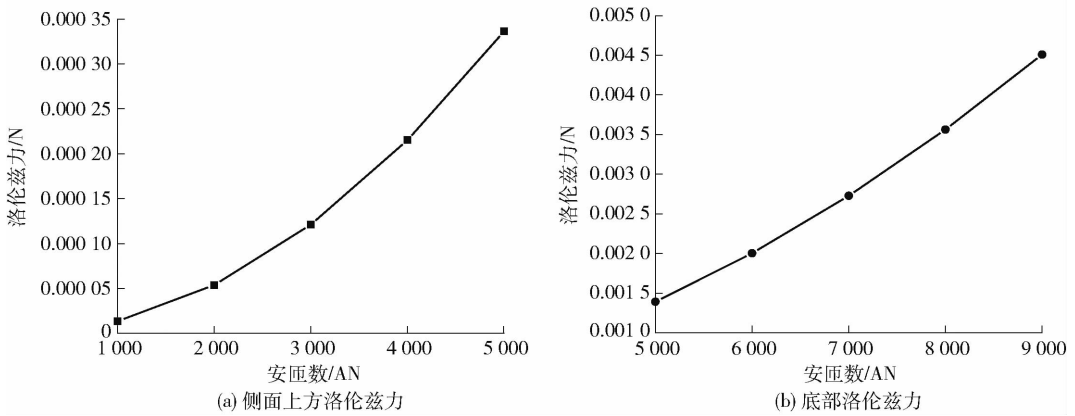
图 10 侧面上方及底部电磁搅拌下槽内最大洛伦兹力点线图
