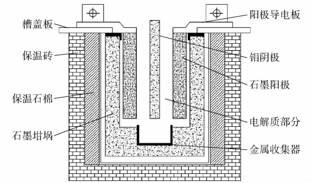
图 1 8 kA 稀土电解槽示意
