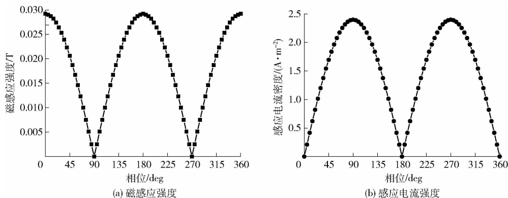
图3 侧面上方线圈 1 Hz/1 000 AN 正弦波电流下槽内最大磁感强度与感应电流强度周期变化
