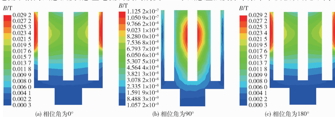
图4 侧面上方线圈 1 Hz/1 000 AN 正弦波电流下槽内磁感强度周期变化云图
