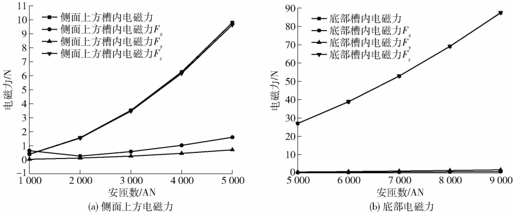
图 11 侧面上方及底部电磁搅拌下槽内最大电磁力点线图
