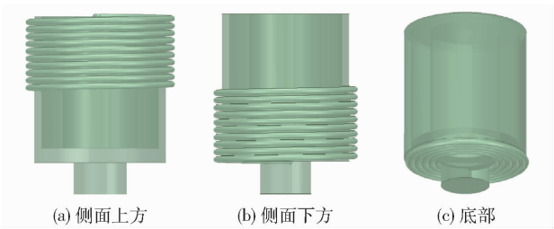
图 2 8 kA 稀土电解槽外加线圈位置
