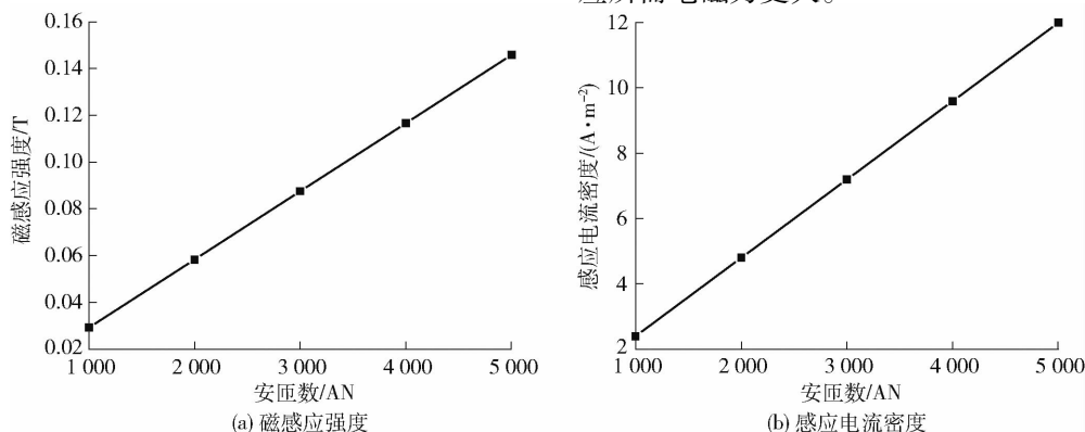
图 8 侧面上方线圈正弦波电流 2 000 ~ 5 000 AN 下槽内最大磁感应强度与感应电流密度点线图
