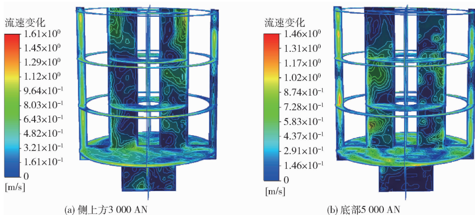
图 13 不同位置对应安匝数电磁搅拌下 20 min 所生成的流场云图
