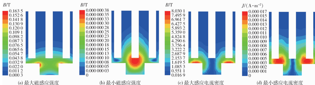
图 7 底部线圈 5 000 AN 下极值磁感应强度与感应电流密度分布云图
