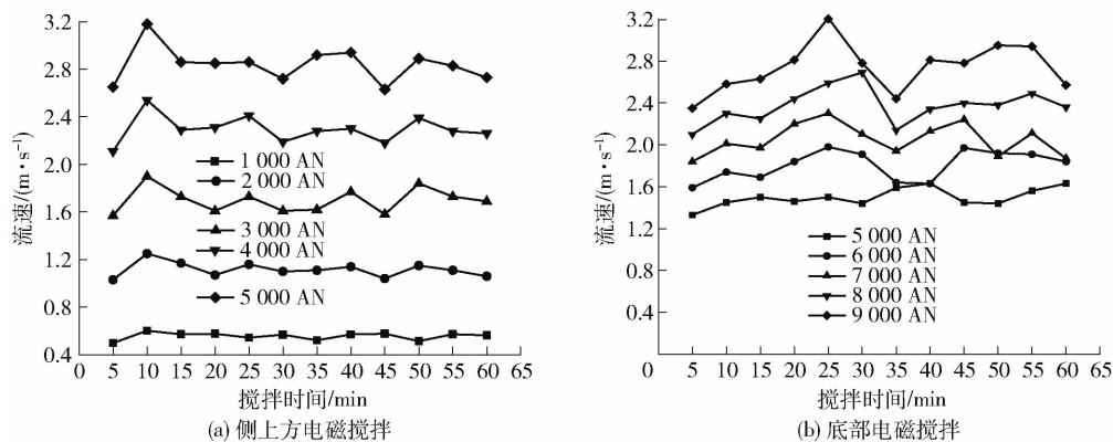
图 12 不同位置电磁搅拌下槽内 1 h 最大流速变化
