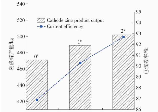
图 12 3 种不同阳极板连续电解 15 d 后的平均锌产量及电流效率
