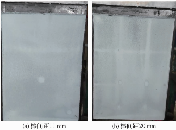
图 14 栅栏型镀膜阳极板棒间距对沉积锌的影响
