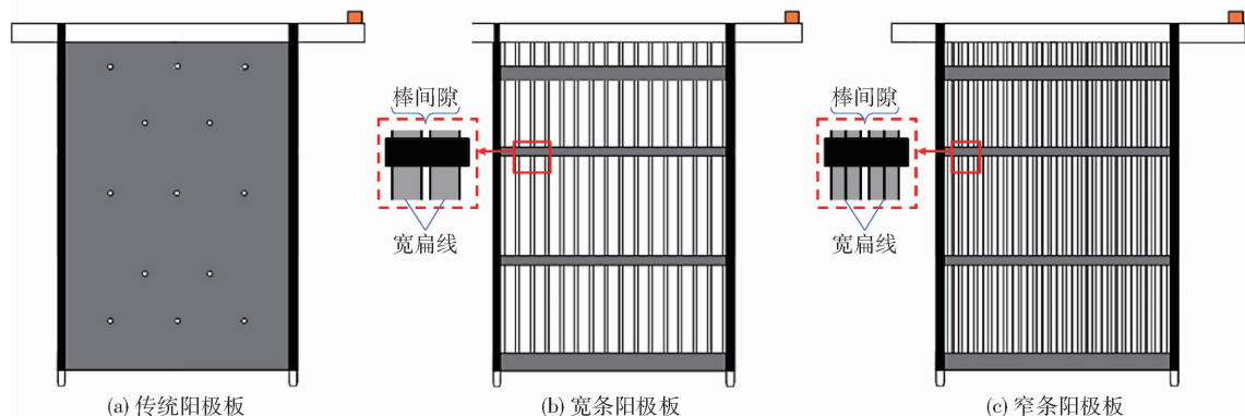
图1 3种不同阳极板型
