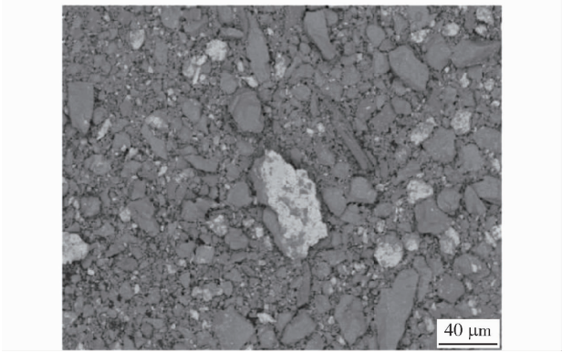
图 6 栅栏型窄条阳极板电解 15 d 后的阳极泥形貌
