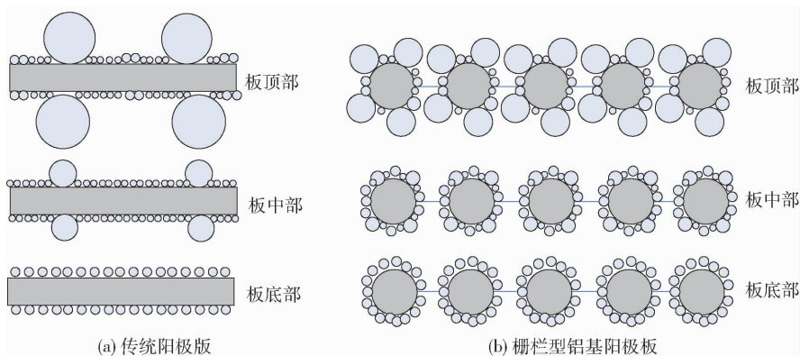
图13 不同阳极板在锌电积过程中的氧气气泡析出状态模型
