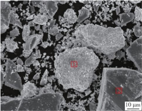
图 7 窄条阳极板表面阳极泥的背散射扫描图
