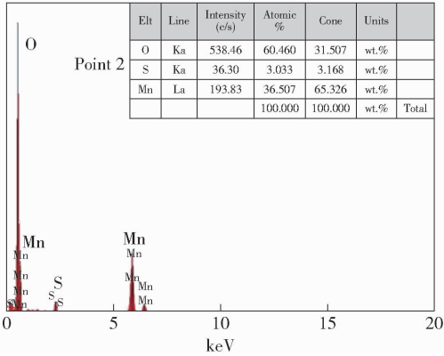
图 9 窄条阳极板表面阳极泥能谱图(点 2)
