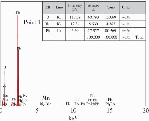
图 8 窄条阳极板表面阳极泥能谱图(点 1)
