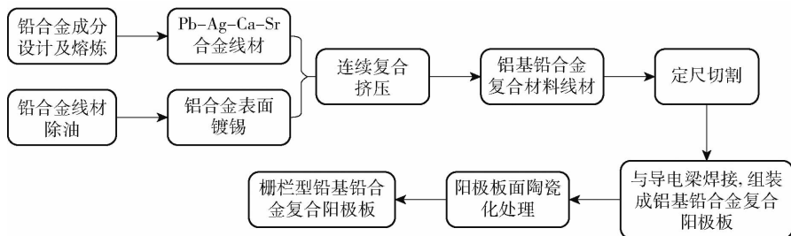
图2 栅栏型铝基铅合金复合阳极板制备工艺流程
