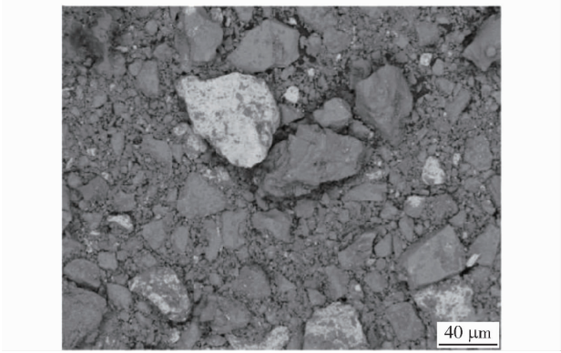
图 5 栅栏型宽条阳极板电解 15 d 后的阳极泥形貌
