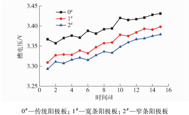
图 11 3 种不同阳极板连续电解 15 d 的槽电压变化
