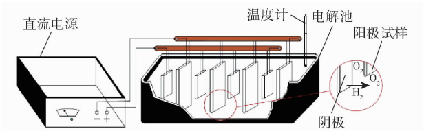
图 3 阳极镀膜装置示意
