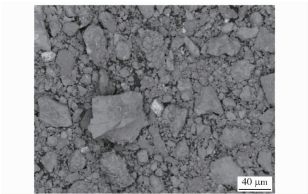
图 4 传统阳极板电解 15 d 后的阳极泥形貌
