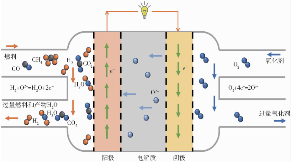
图1 固体氧化物燃料电池原理示意
