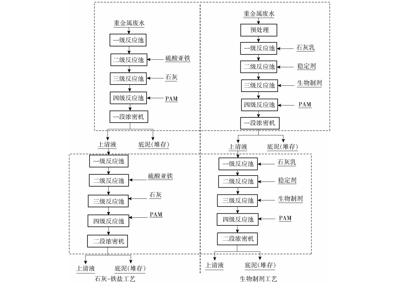
图1 石灰-铁盐工艺流程和生物制剂深度处理协同脱铊工艺流程
