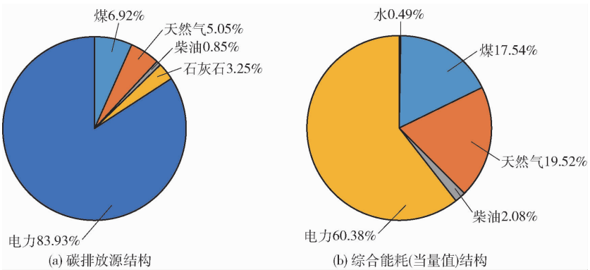
图1 按区域电网排放因子核算的碳排放与按当量值核算的综合能耗结构对比
