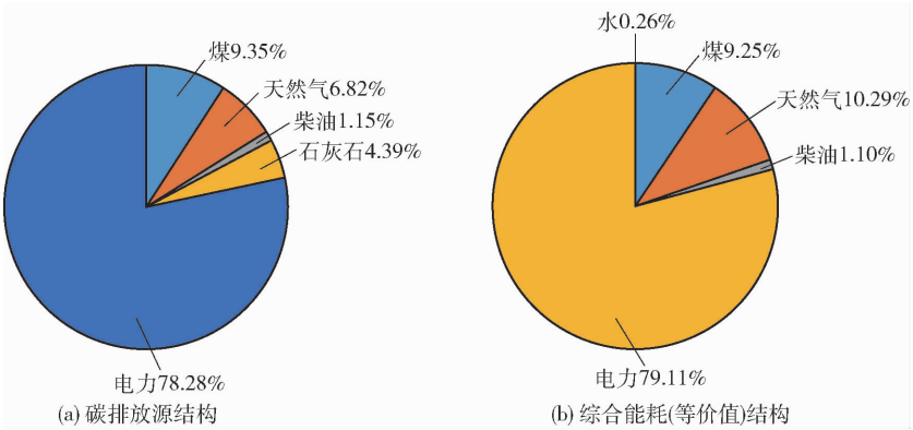
图2 按全国电网排放因子核算的碳排放与按等价值核算的综合能耗结构对比
