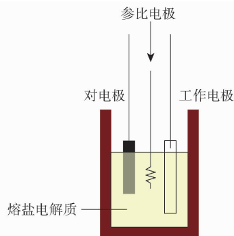
图 1 电化学实验电解槽示意图
