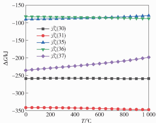
图 2 反应式(30)~(31)和反应式(35)~(37)的 \Delta G 与 T 的关系
