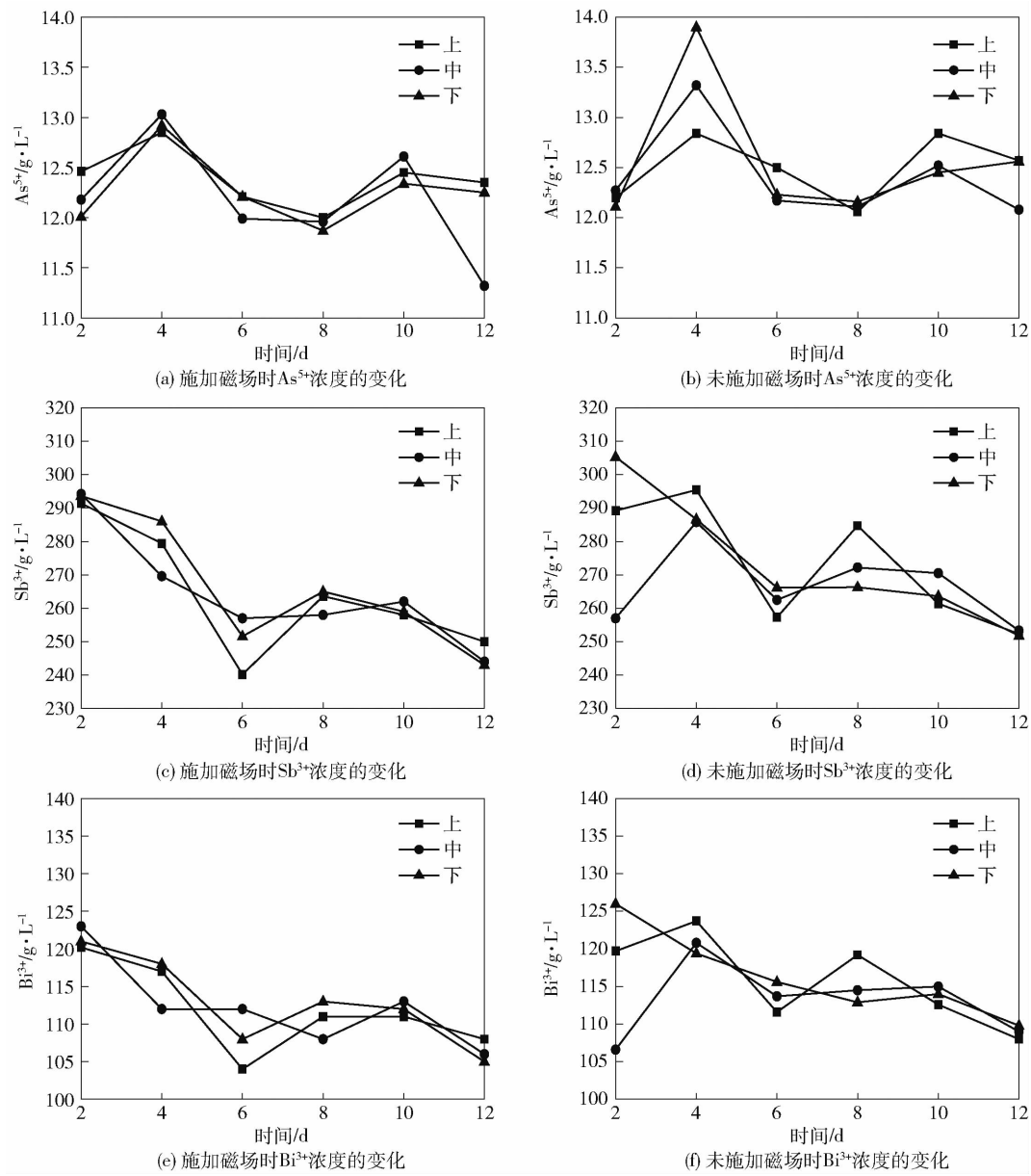
图3 磁场对电解液中 As 5+ 、Sb 3+ 和 Bi 3+ 浓度的影响
