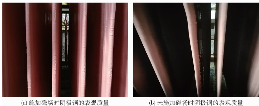
图5 磁场对阴极铜表观质量的影响
