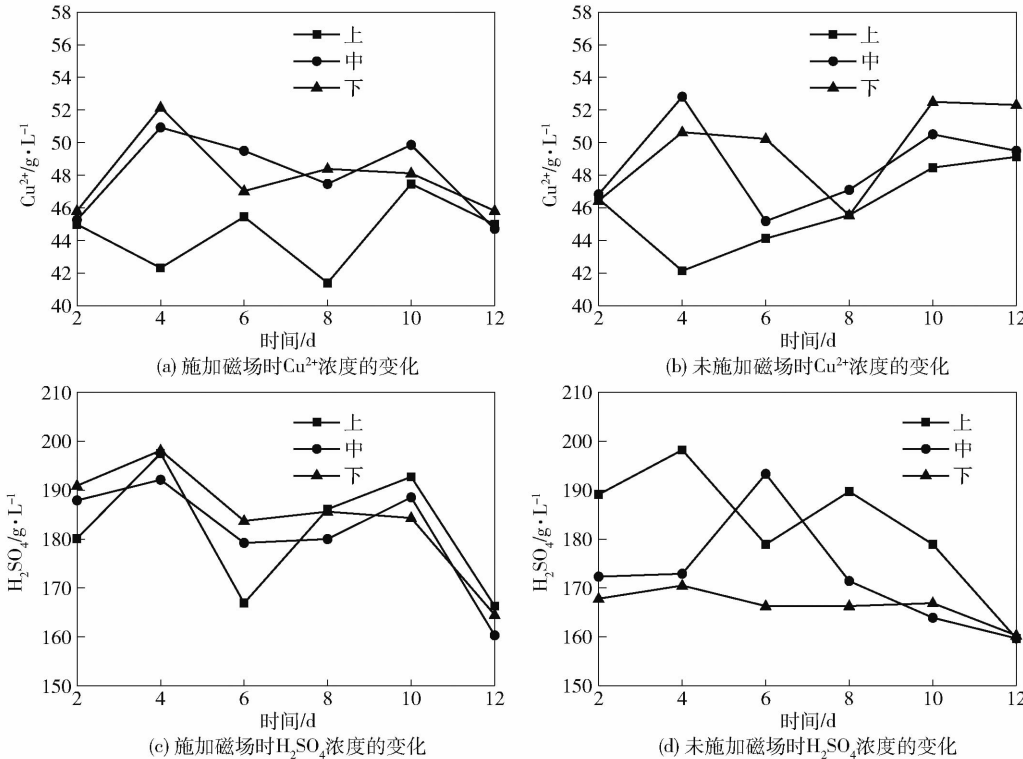
图 2 磁场对 Cu 2+ 和 H 2 SO 4 浓度的影响
