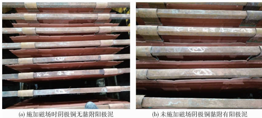
图4 磁场对阴极铜黏附阳极泥情况的影响
