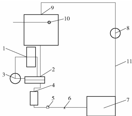
1—磁场; 2—过渡槽; 3—1号循环泵; 4—电解槽; 5—流量计; 6—阀门; 7—低位槽; 8—2号循环泵; 9—高位槽; 10—蒸汽加热装置; 11—管道
