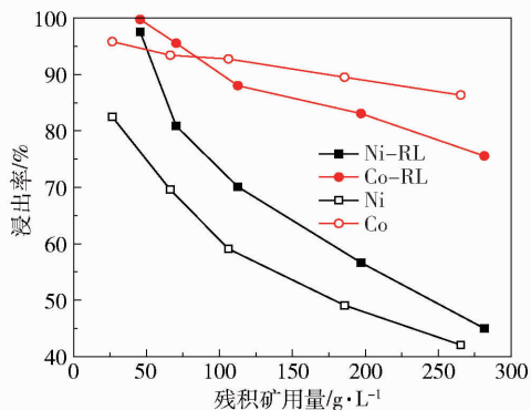
图3 还原浸出、常规浸出镍钴浸出率及终点酸度对比
