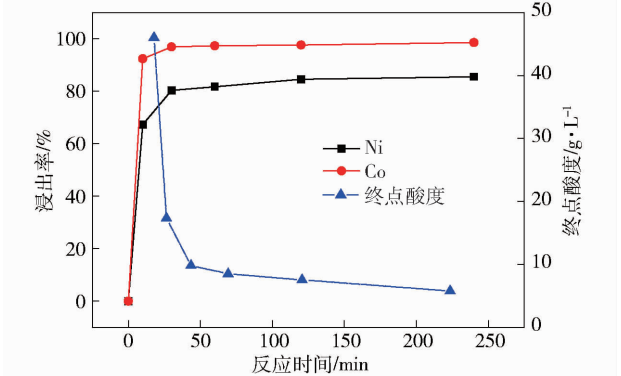
图 2 反应时间对镍钴浸出率及终点酸度的影响
