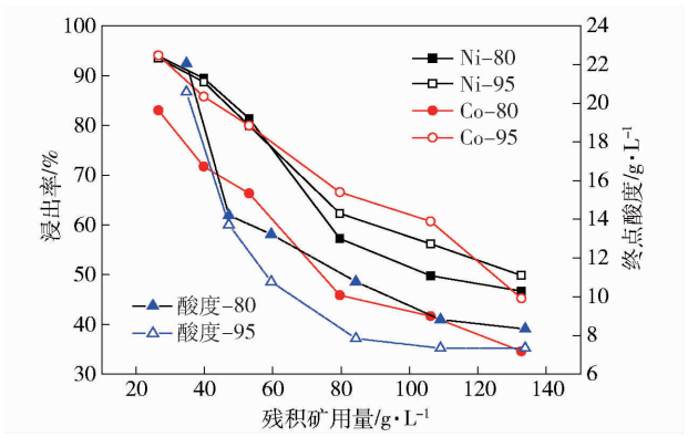
图 1 磨矿细度、残积矿用量对镍钴浸出率及终点酸度的影响
